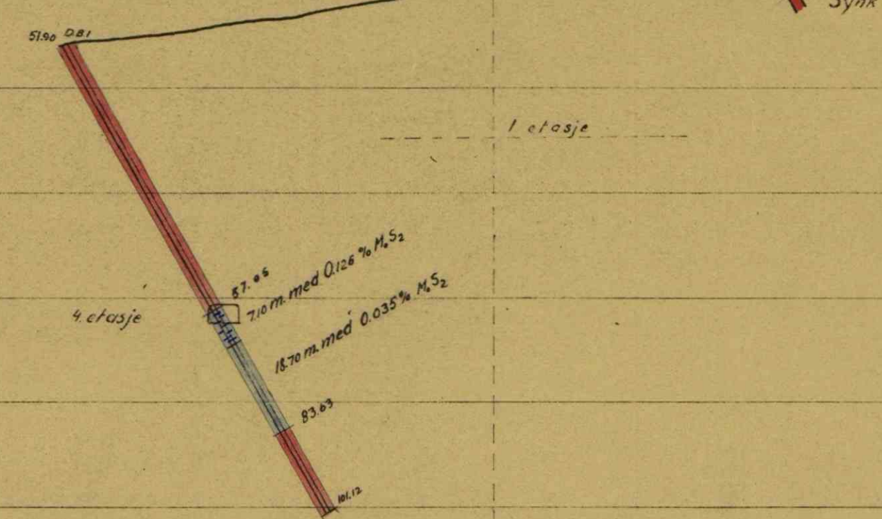
BORRPROFIL 1 (GRUBEPROFIL 26)
