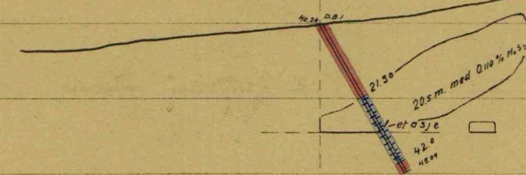
BORRPROFIL 2 (GRUBEPROFIL 28)
