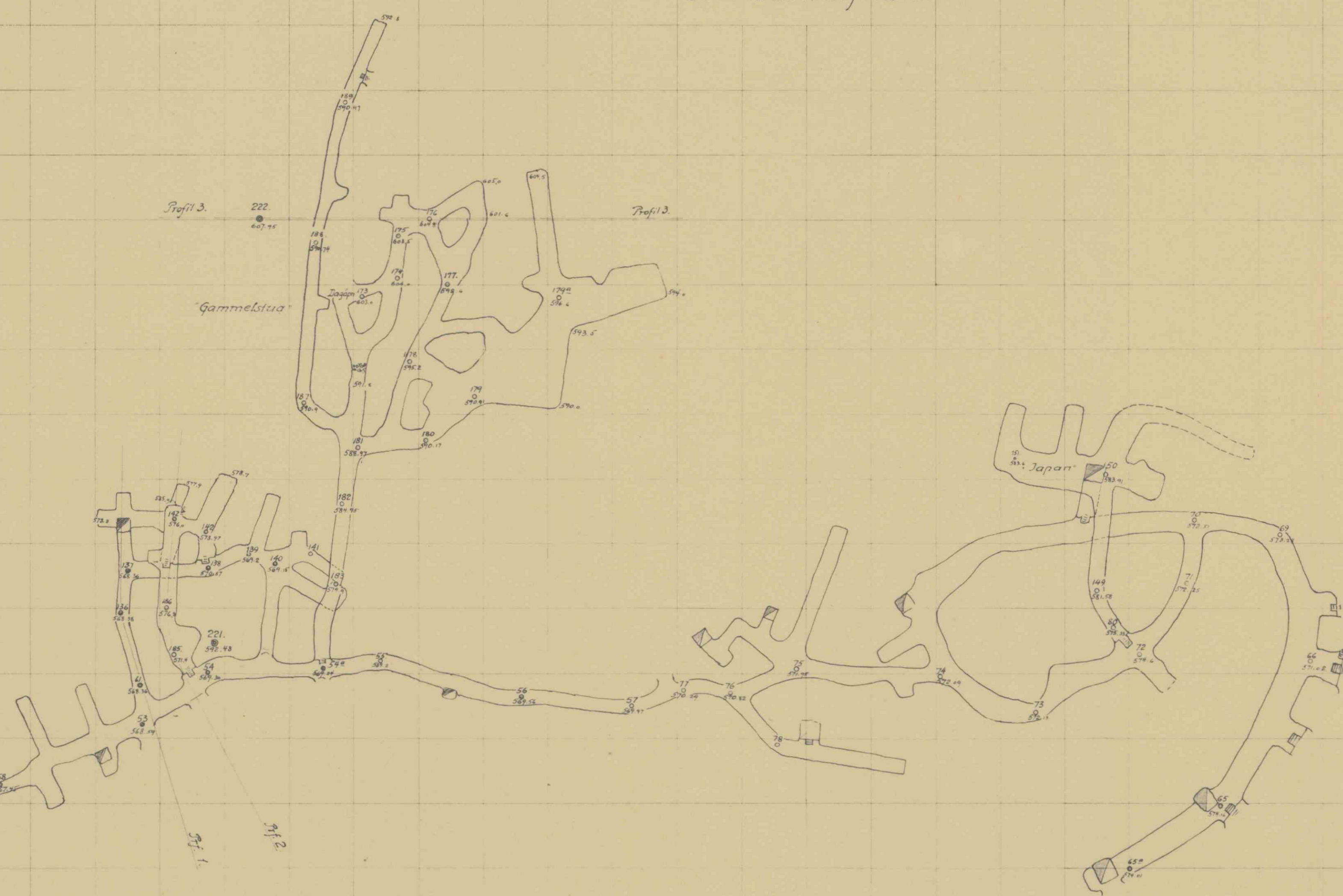
Horisontalsplan.
