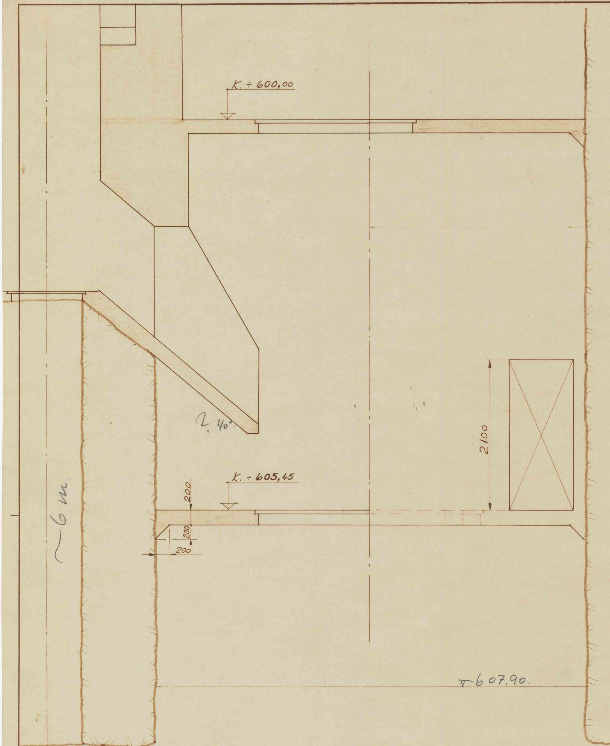
Snitt A-A
