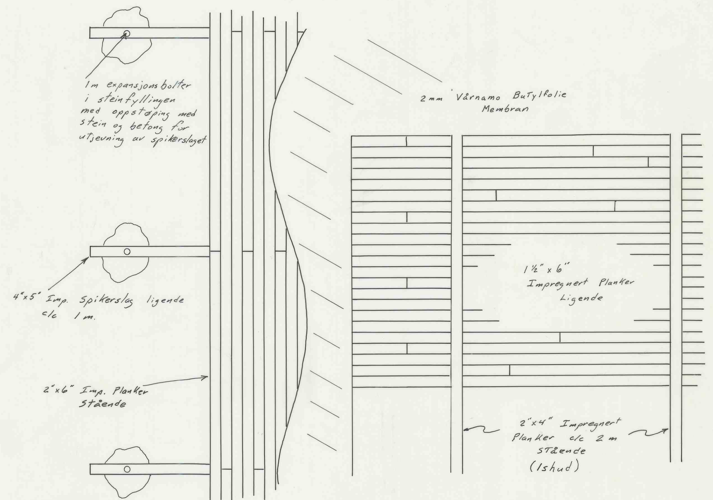
DETALJER OM PLANKEDEKKET 1:10
