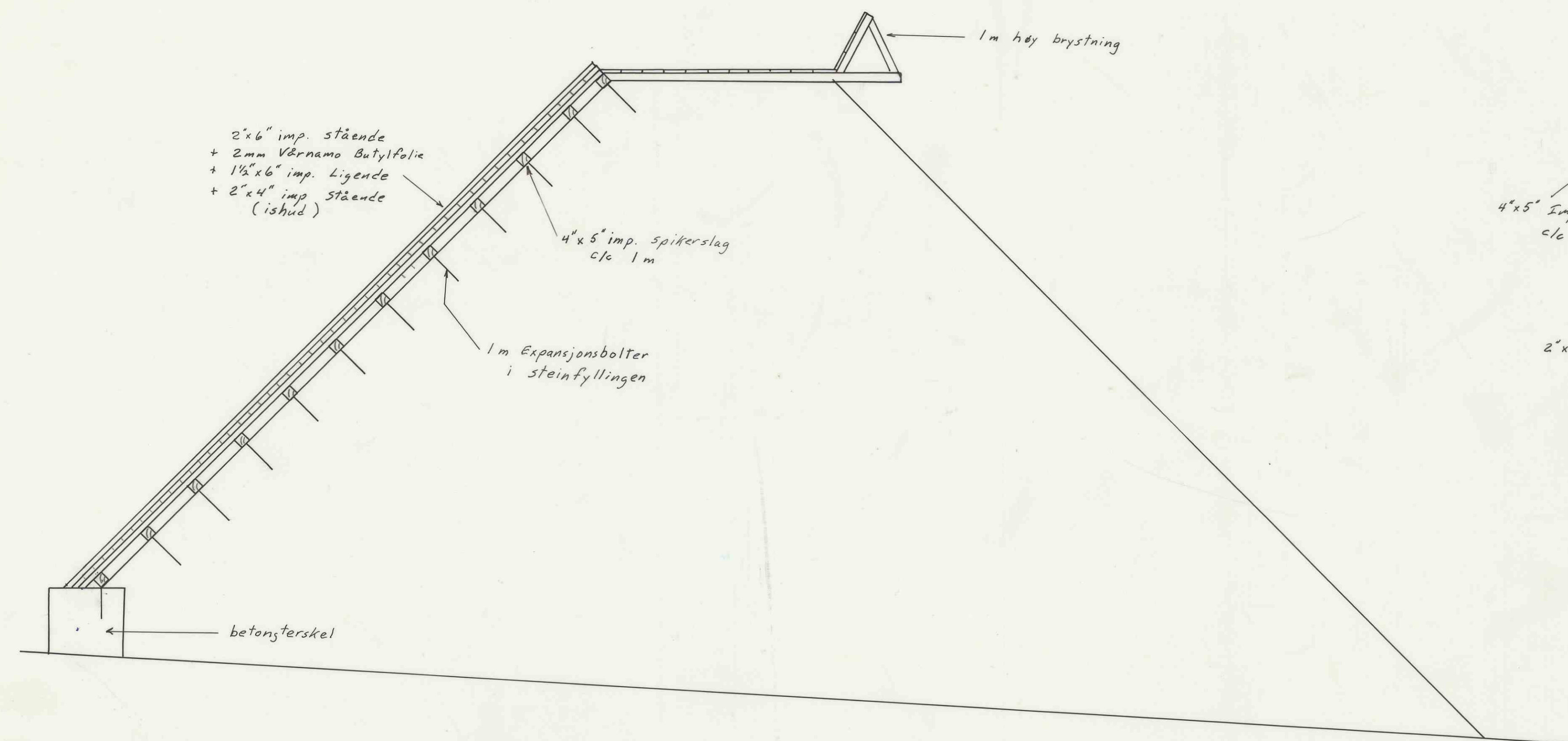
SNITT A - A 1:50
