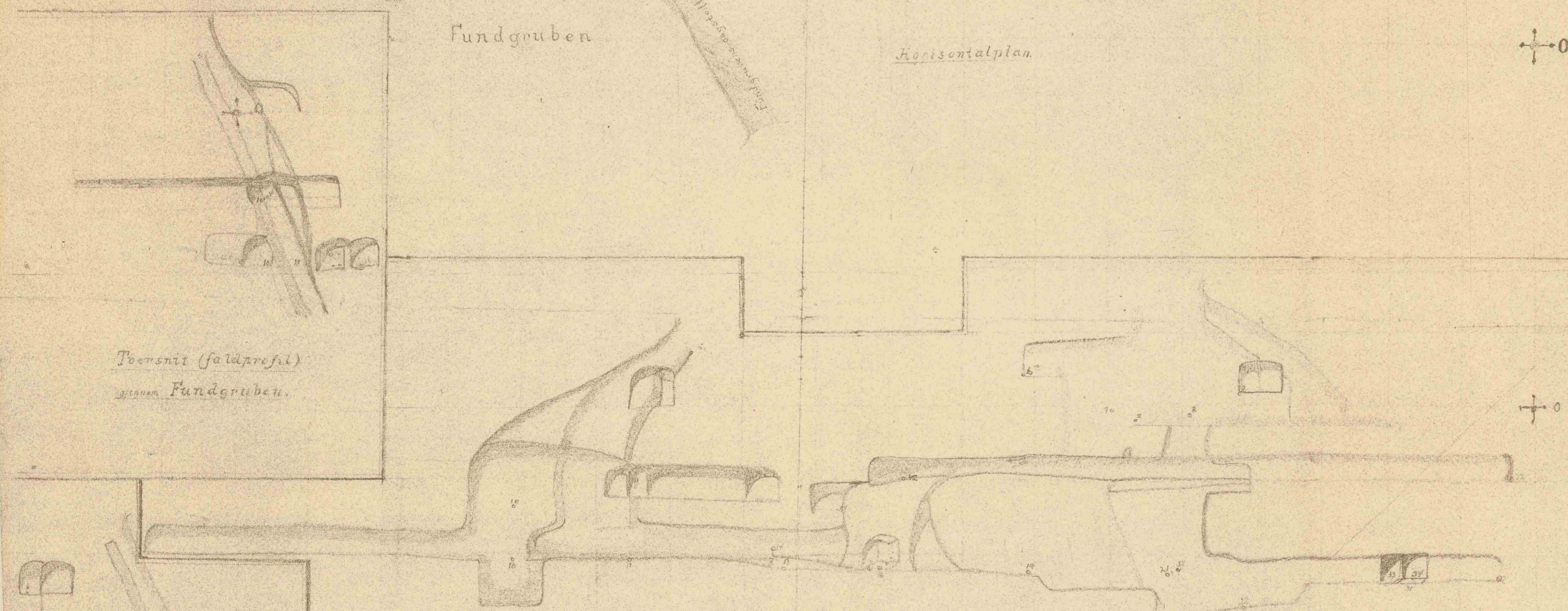
Langdesnit (feltprofil) gjennem Fundgruben og Storgruben.
