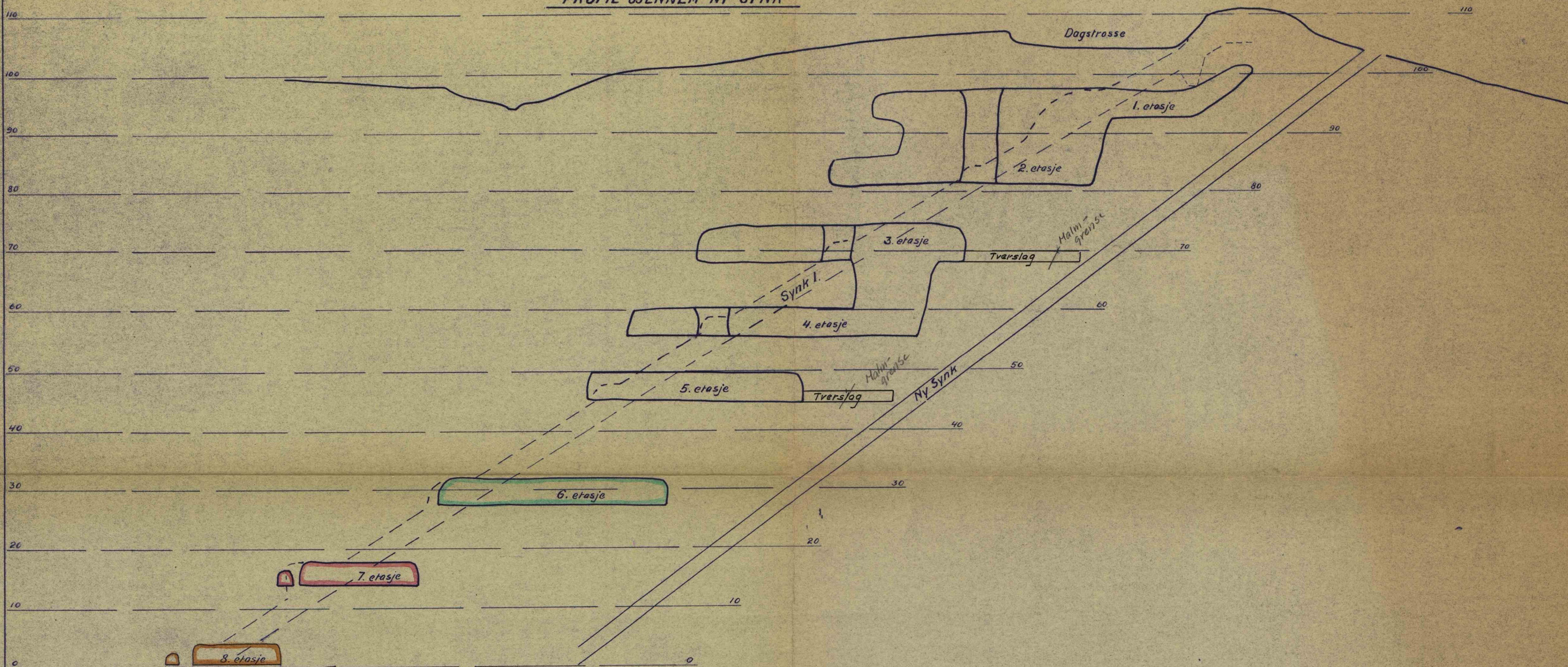
NIVÅKART OVER 6, 7 og 8. ETASJE
