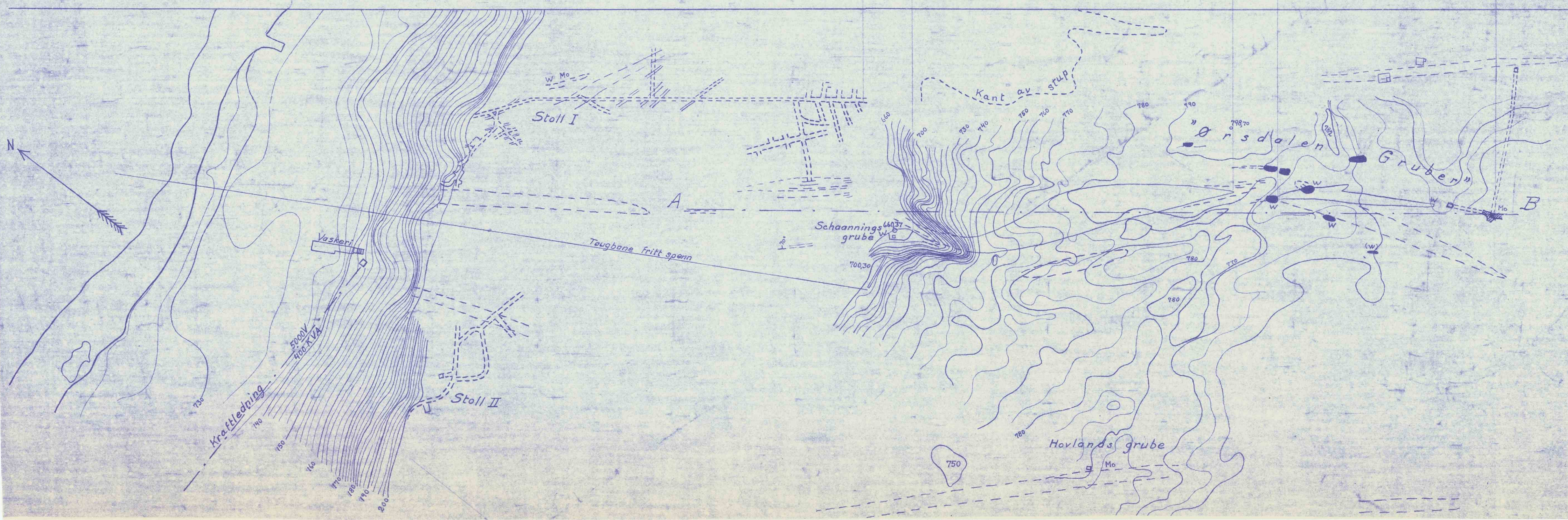
Profil A - B Aplittlinser, malmforekomster, stoller og synken.
