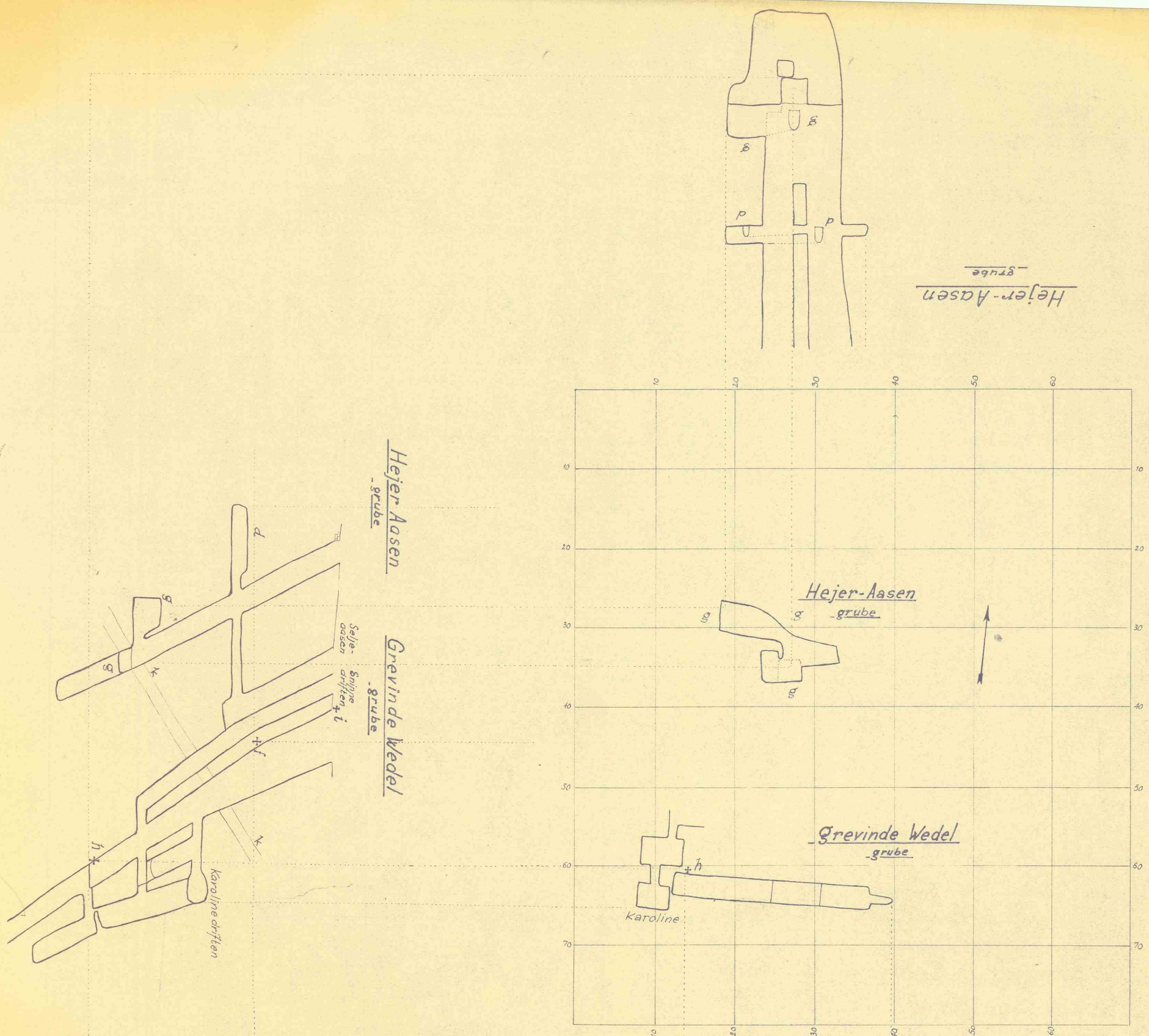
Grundtegning af de i drift værende Solberg- grubers nederste dyp.
