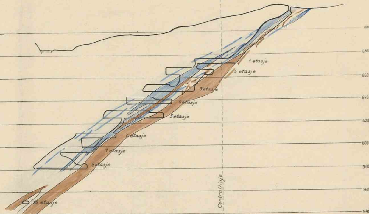
PROFIL 20
