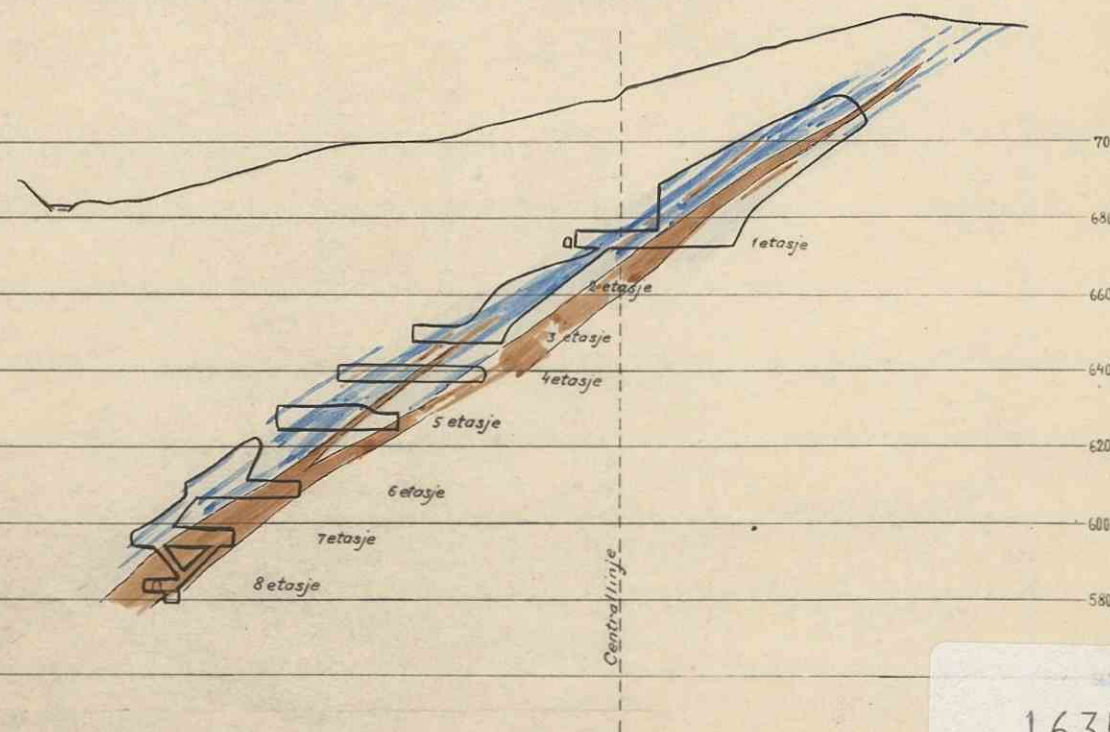
PROFIL 22
