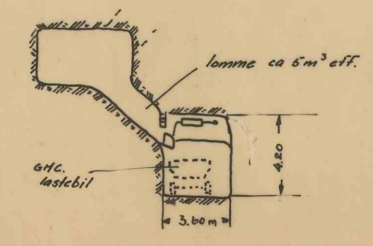
Snitt B-B
