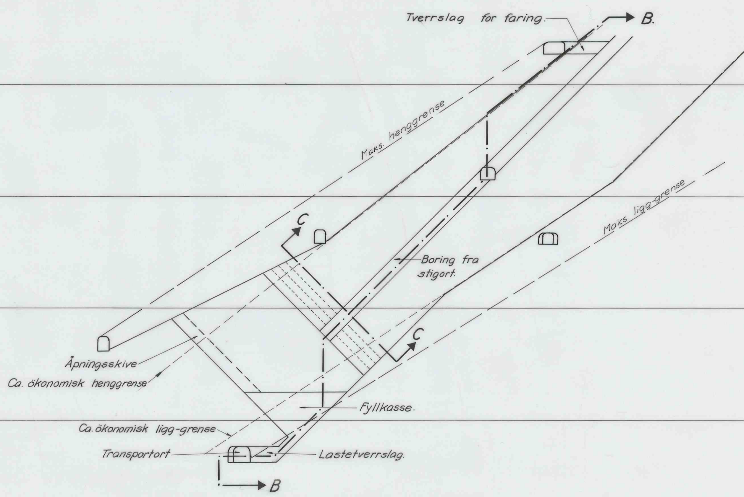
Snitt A-A.
