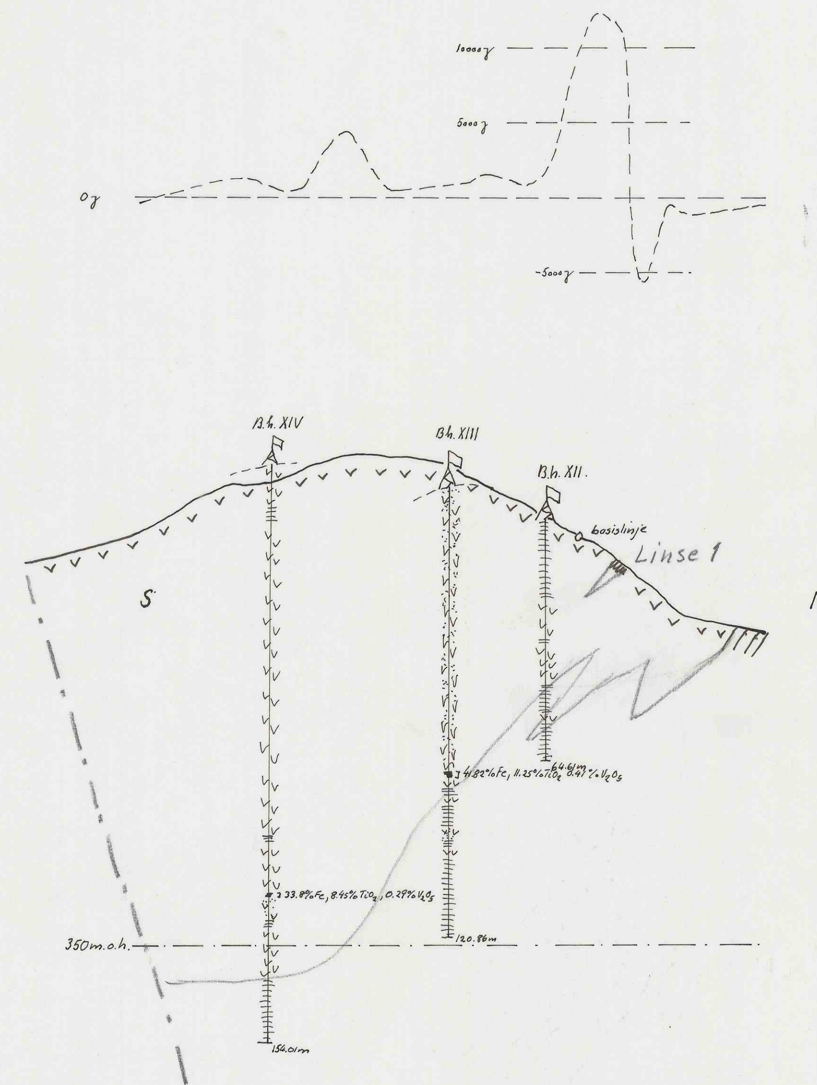
Profil 5V.
