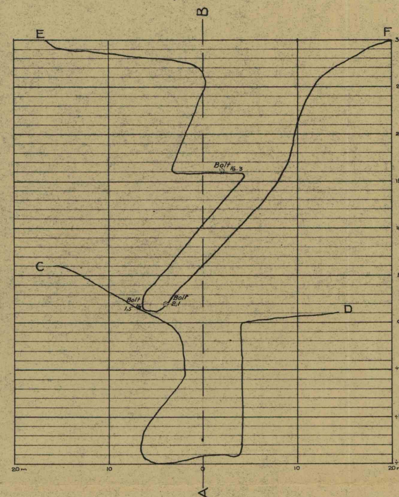
Tverrprofiler 1:250
