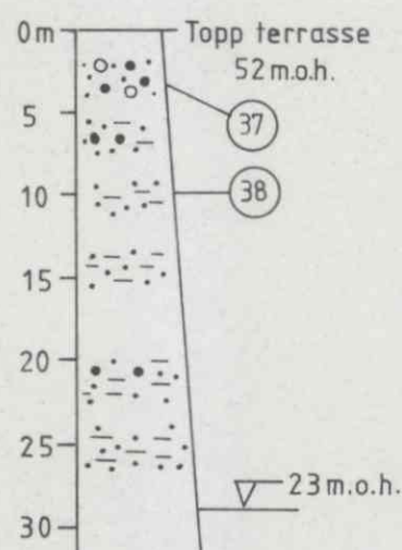
Snitt B
