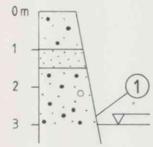
Snitt A
