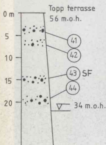
Snitt D
