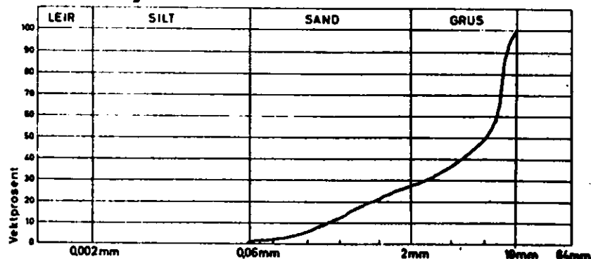
Kornfordelingskurve
