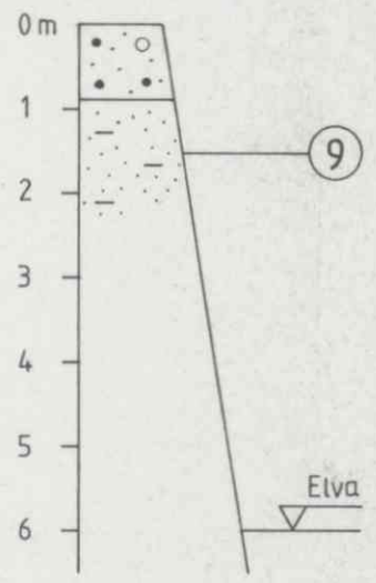
Snitt G
