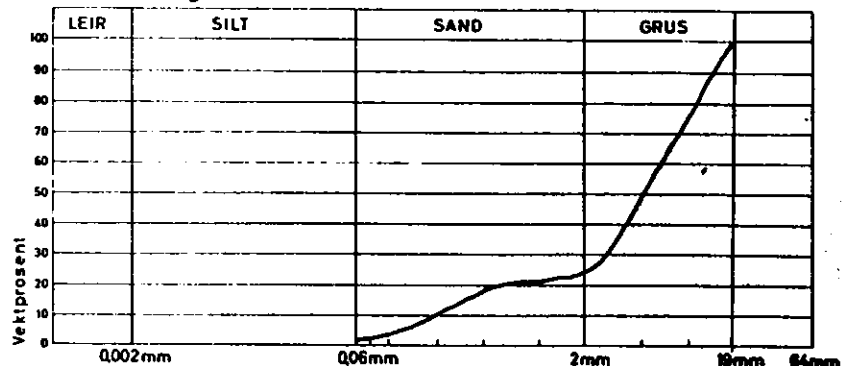
Kornfordelingskurve
