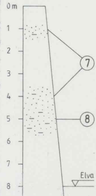
Snitt F
