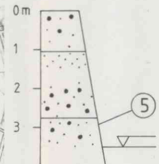
Snitt D
