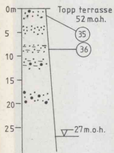
Snitt A
