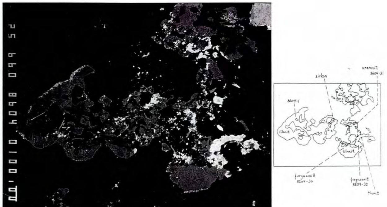
Fig. 42. Back-scatterbilde av titanitt, zirkon og fergusonitt med inneslutninger av uraninit. Ett thorittkorn er innesluttet i biotitt. Skalastreken er 100 \mu m.
