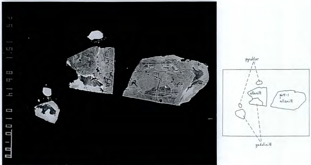
Fig. 36. Back-scatterbilde av allanitt, gadolinitt og pyrochlor. Skalastreken er 100 \mu\text{m} .
