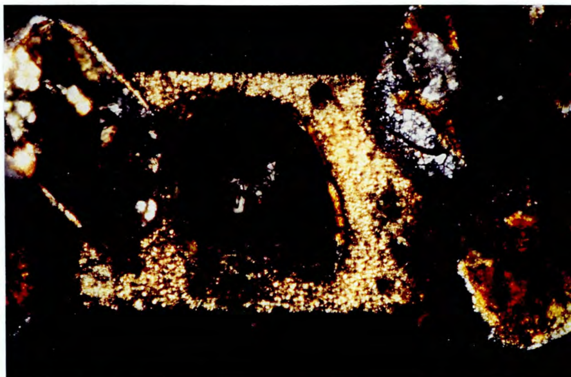
Fig. 16. Sonert gadolinitt med kvartsinneslutninger, fra mineralkonsentrat. a, upolarisert lys - b, X nicoll. De to brungule kornene nederst er pyroklor. De to andre er thoritt. Skalastreken er 100 \mu\text{m} .
