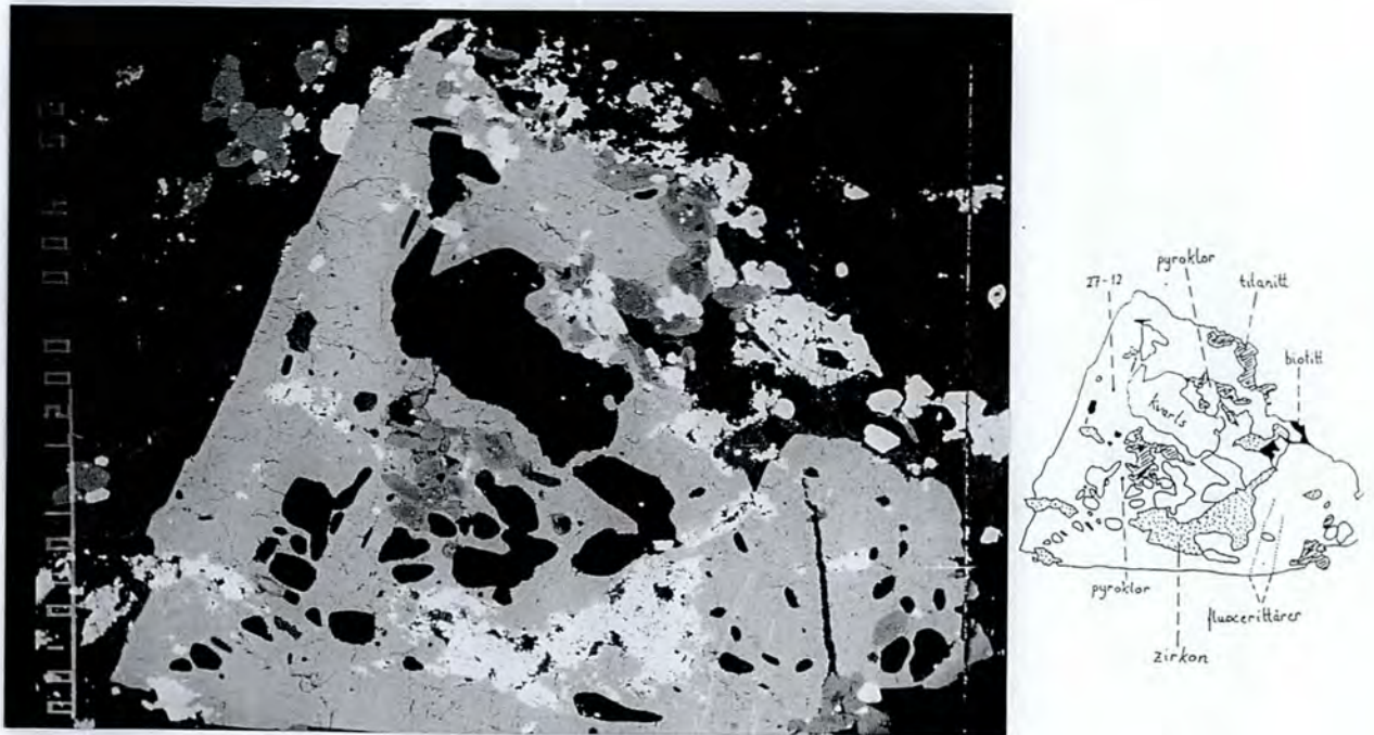
Fig. 29. Back-scatterbilde av genthelvinkrystall med inneslutninger av titanitt (skravert), zirkon (prikkraster), biotitt (svart), pyroklor, kvarts og feltspat (svarte på back-scatterbildet) og fluocerittårer. Skalastreken er 1 mm.
