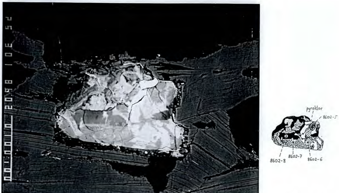
Fig. 89. Back-scatterbilde av fler-faset LREE-mineral innesluttet i biotitt og med pyrochlor-inneslutning. Skalastreken er 100 \mu\text{m} .
