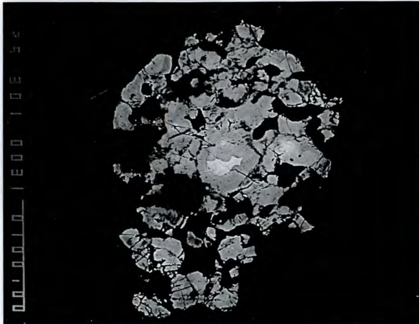
Fig. 47. Back-scatterbilde av pyroklor. Analyse nr. 31-10a og 31-10b er fra henholdsvis lys og mørk fase. Skalastreken er 100 \mu\text{m} .
