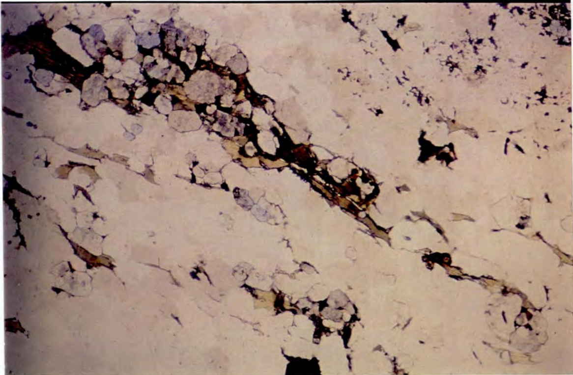
Fig. 4. Typisk fenakittmalm. Foruten fenakitt (korn med høyt relieff) er det biotitt, zirkon (øverste høyre hjørne), kvarts og feltspat. Upolarisert lys. Skalastreken er 100 \mu\text{m} .
