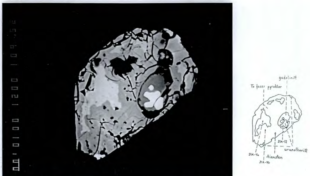
Fig. 26. Back-scatterbilde fra mineralkonsentrat av to-faset pyroklor med inneslutning av gadolinit som igjen inneslutter uranothoritt. Ett tinnstenkorn er også innesluttet i pyrokloren. Skalastreken er 10 µm.
