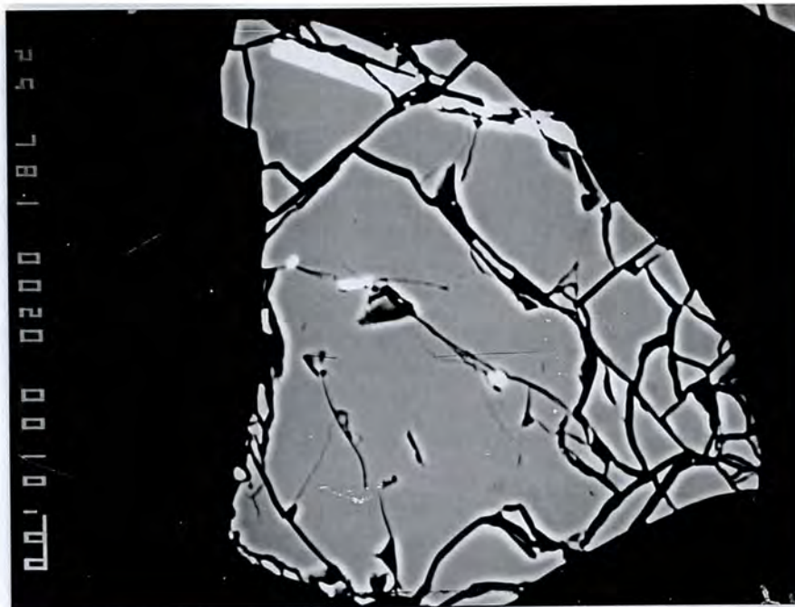
Fig. 78. Back-scatterbilde fra mineralkonsentrat av magnetitt med innslutninger av fergusonitt. Skalastreken er 10 µm.
