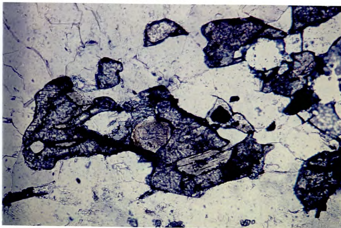
Fig. 82. Kainositt og thalenitt innesluttet i titanitt. Upolarisert lys.
