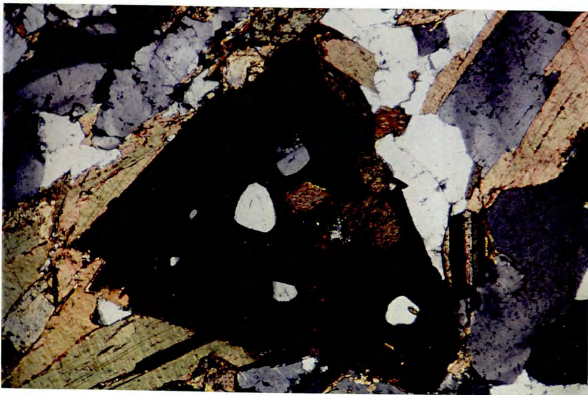
Fig. 30. Genthelvin ved upolarisert lys (a) og X nicoll (b). Foruten kvarts og feltspat er det også biotitt (grønn) og titanitt. Skalastreken er 100 \mu m.
