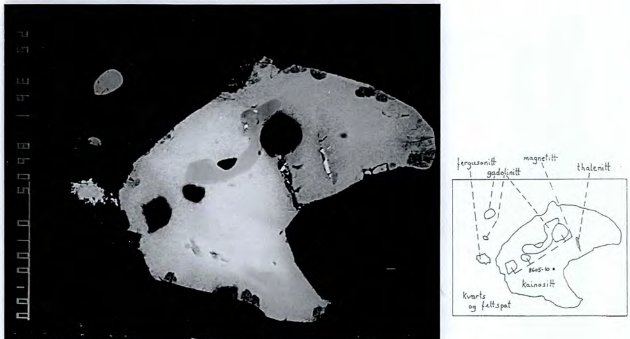
Fig. 25. Back-scatterbilde av kinositt med inneslutninger av gadolinit, thalenit og magnetit. Skalastreken er 100 µm.
