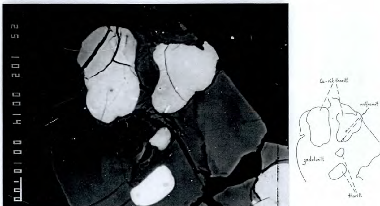
Fig. 93. Back-scatterbilde fra mineralkonsentrat av wolframitt innesluttet i thoritt som er omgitt av gadolinitt. Skalastreken er 10 \mu\text{m} .
