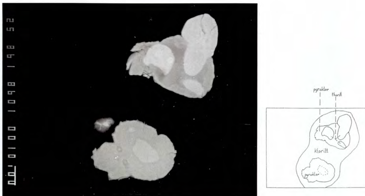
Fig. 51. Back-scatterbilde av pyrochlor og thoritt med påvokst randfase av kloritt. Skalastreken er 10 \mu\text{m} .
