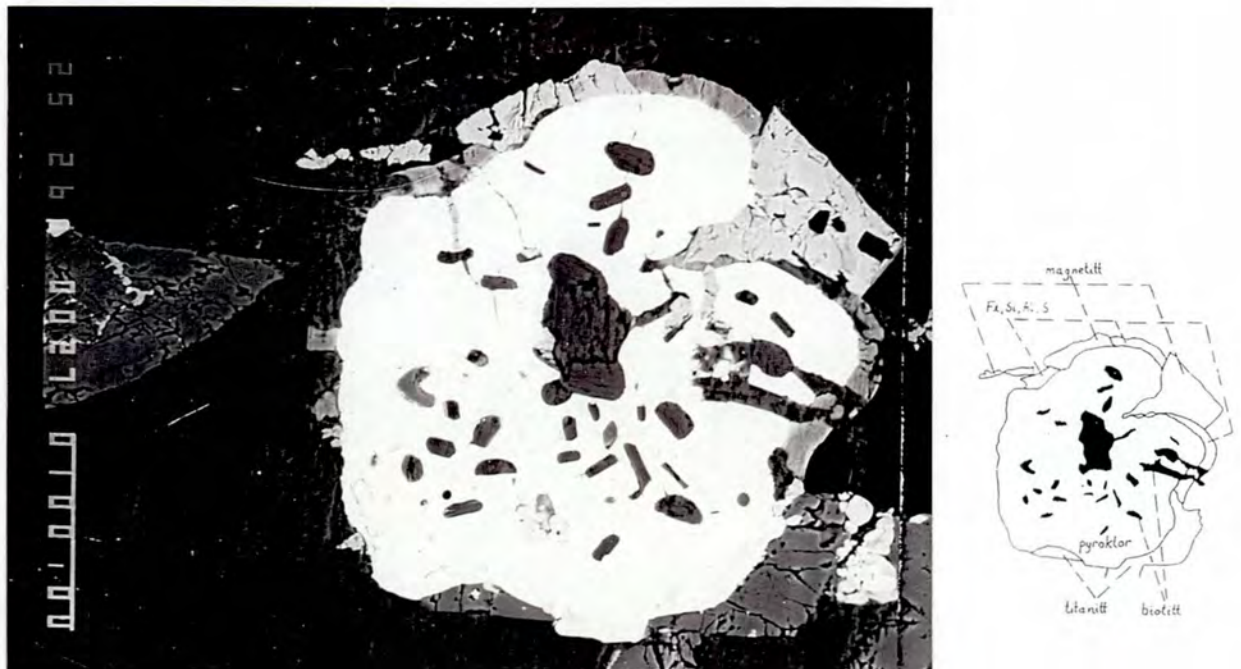
Fig. 49. Back-scatterbilde av pyrochlor med biotittinneslutninger og rand-sone av magnetitt og en Fe-Si-Al-S-fase. Skalastreken er 100 \mu\text{m} .
