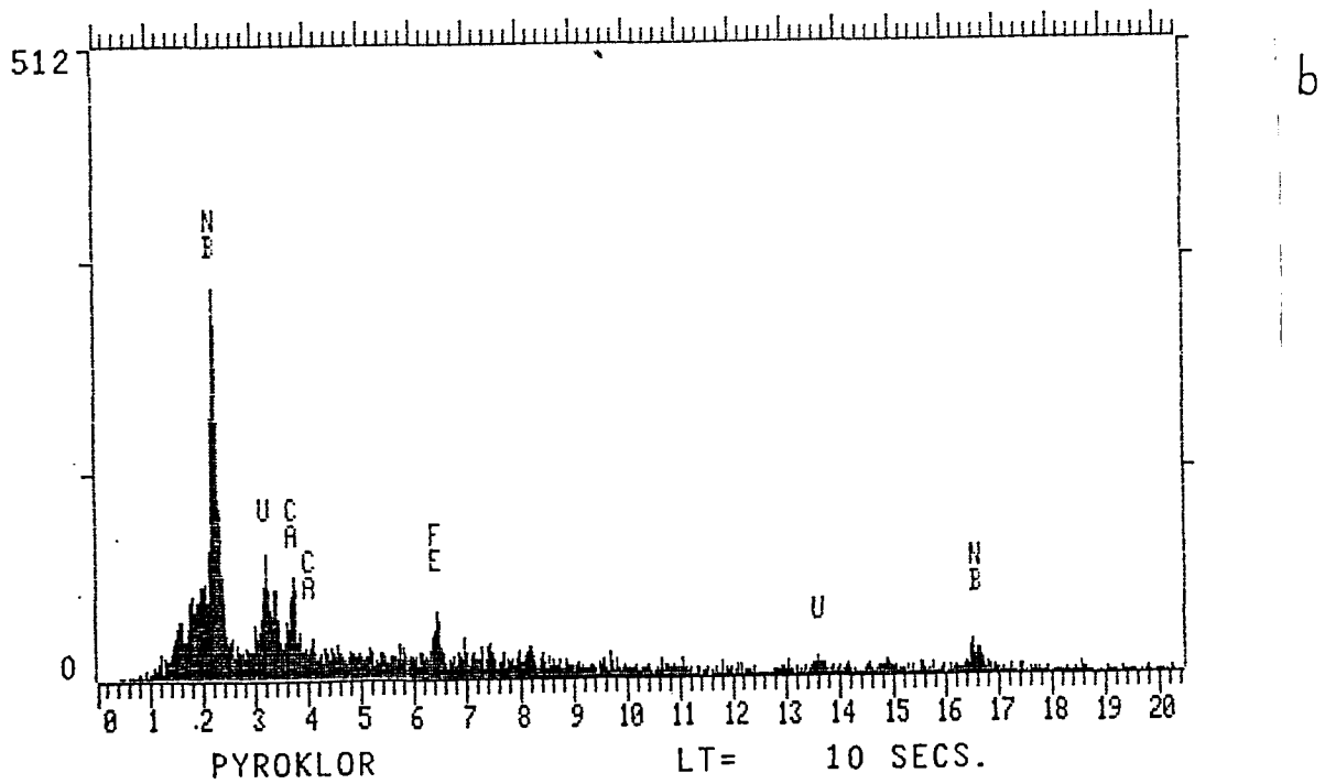
Fig. 55. EDS-spekter av pyrochlor. a, er lys fase og b, er mørk fase.
