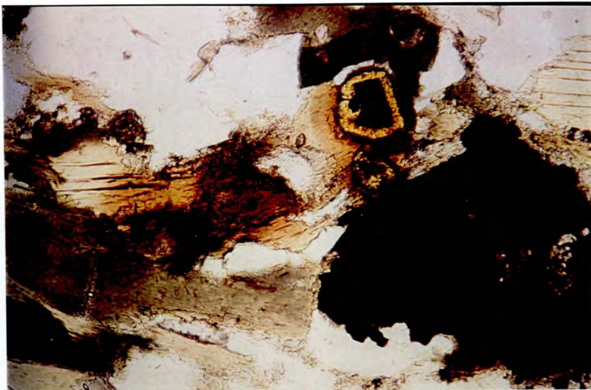
Fig. 54. Pyroklor. 3 korn midt på bildet: to gule med opak kjerne og ett rødbrunt. (Se også fig. 56). Ellers er det kvarts, feltspat, biotitt, zirkon og magnetitt (det store opake til høyre). Upolarisert lys. Skalastreken er 100 \mu\text{m} .
