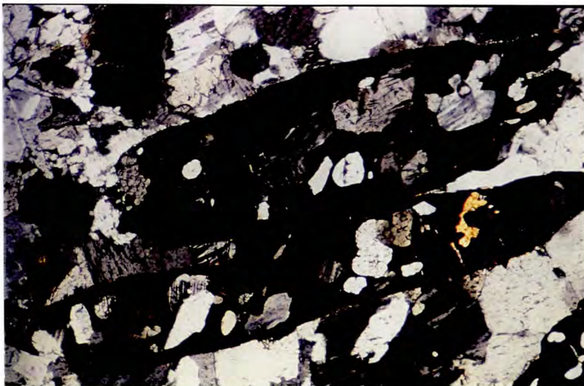
Fig. 9. Be-rhönitt (svart) med inneslutninger av fenakitt (gult), kvarts og feltspat. x nicoll. Skalastreken er 100 \mu\text{m} .
