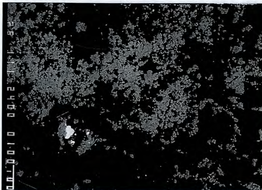
Fig. 58. Back-scatterbilde av zirkonsky. Hvite korn nederst til venstre er thoritt. Skalastreken er 100 \mu\text{m} .
