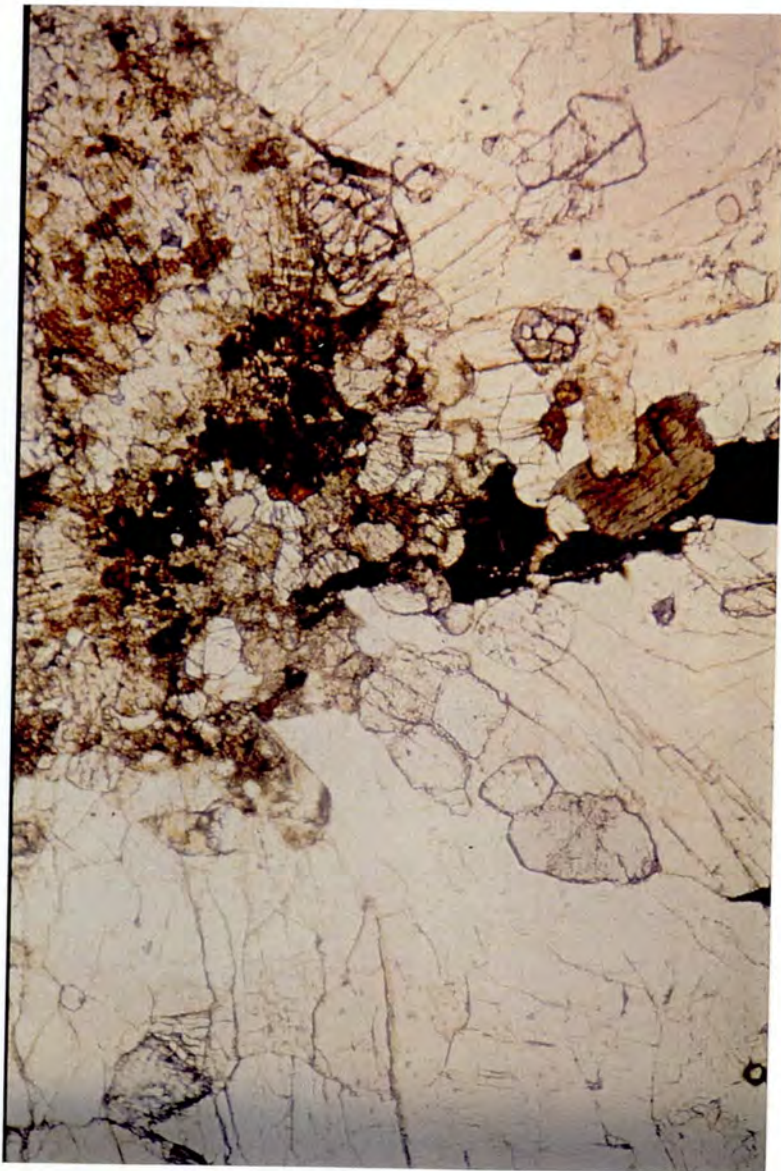
Fig. 33. Allanitt (brun) som omslutter pyroklor, thoritt, fenakitt, apatitt, gadolinitt og blyglans. Upolarisert lys. Back-scatterbilde med forklaring av samme aggregat i fig. 34. Skalastreken er 100 \mu\text{m} .
