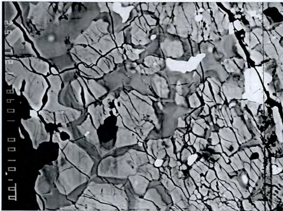
Fig. 38. Back-scatterbilde av to-faset allanitt (utsnitt fra fig. 34) med inneslutninger av gadolinitt. Analyse nr. 8601-11 og 8601-12 er fra henholdsvis lys og mørk fase. Skalastreken er 10 \mu m.
