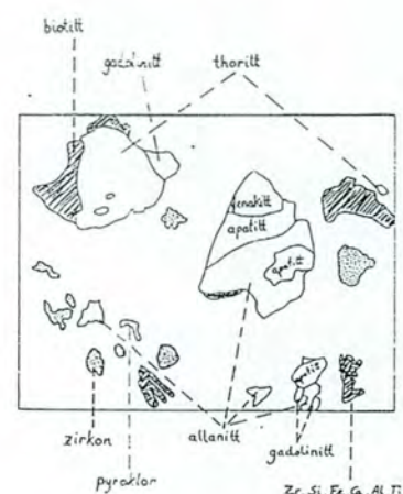
Fig. 8. Katodeluminisens-bilde (a) fra mineralkonsentrat. b er back-scatter-bilde av samme utsnitt og viser thoritt, gadolinitt, pyroklor, apatitt, allanitt, zirkon (prikkraster), biotitt (skravert) og fenakitt. Skalastreken er 100 \mu m.
