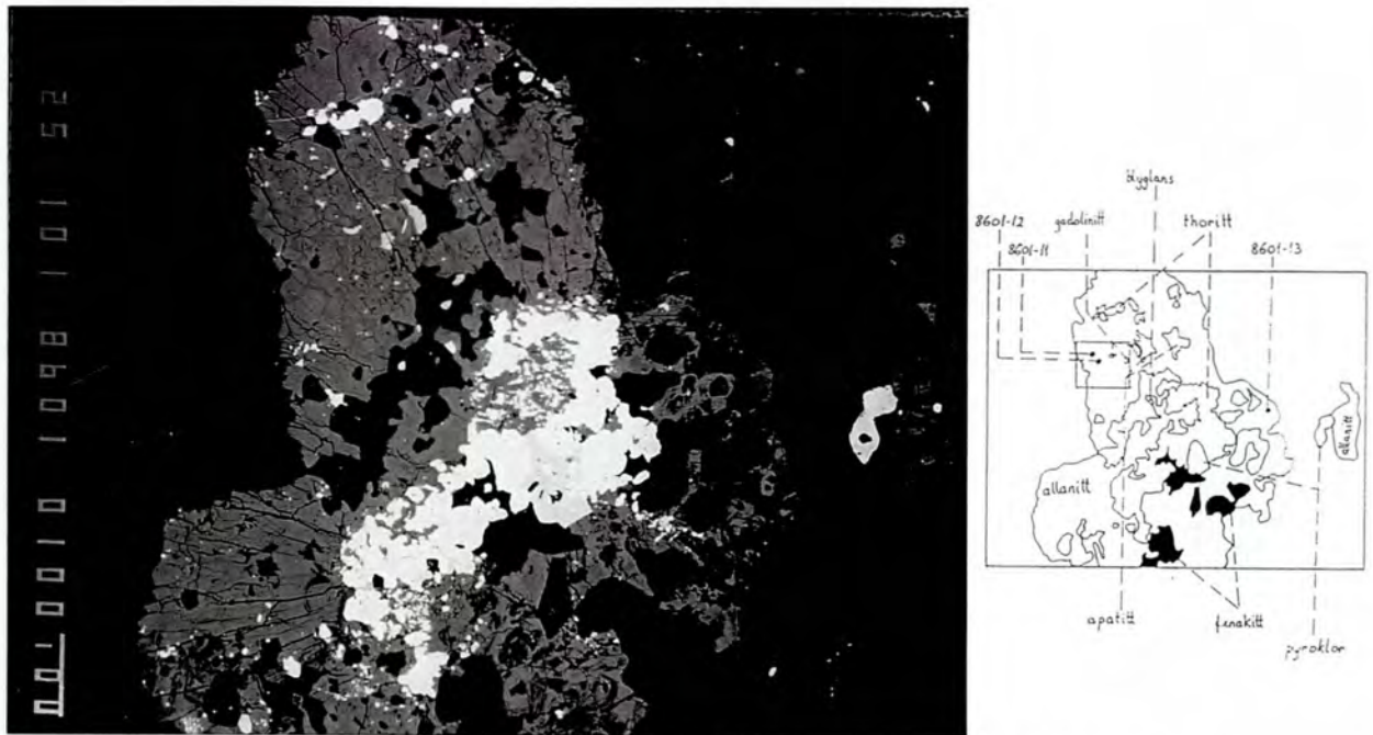
Fig. 34. Back-scatterbilde av allanitt (forstørret utsnitt i fig. 38) som omslutter pyroklor, thoritt, fenakitt, apatitt, gadolinitt og blyglans. Skalastreken er 100 \mu m.
