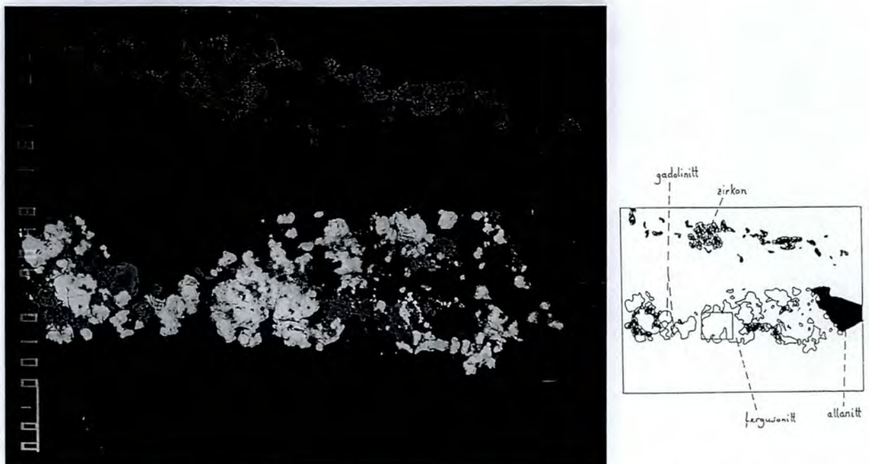
Fig. 79. Back-scatterbilde av fergusonitt (lyse grå), gadolinit, zirkon (skravert) og allanitt (svart). Skalastreken er 100 µm.
