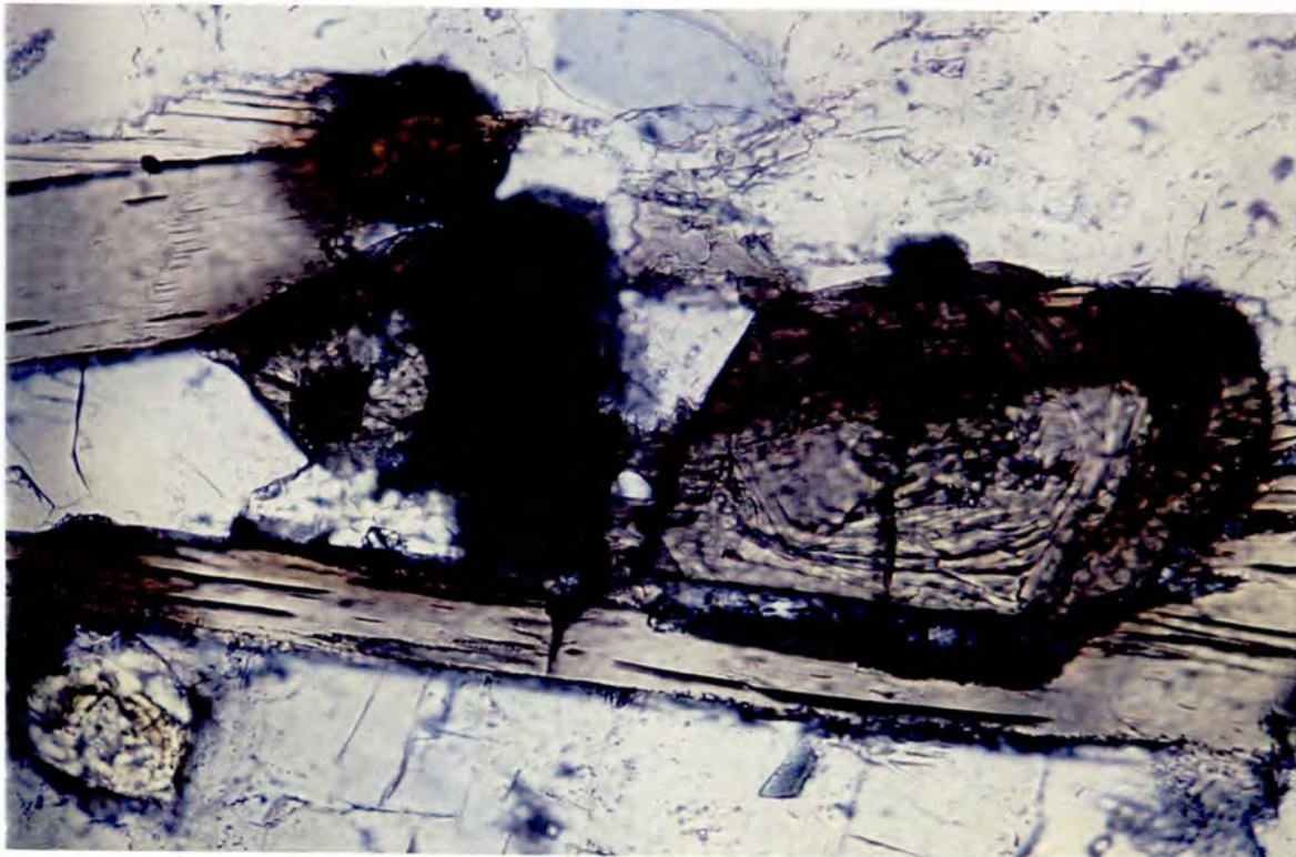
Fig. 35. Allanitt, gadolinitt og pyroklor. Forklaring i fig. 36 som er back-scatterbilde av de samme korn. Upolarisert lys. Skalastreken er 100 \mu m.
