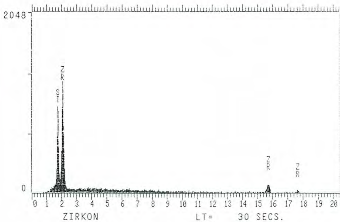
Fig. 63. EDS-spekter av zirkon.
