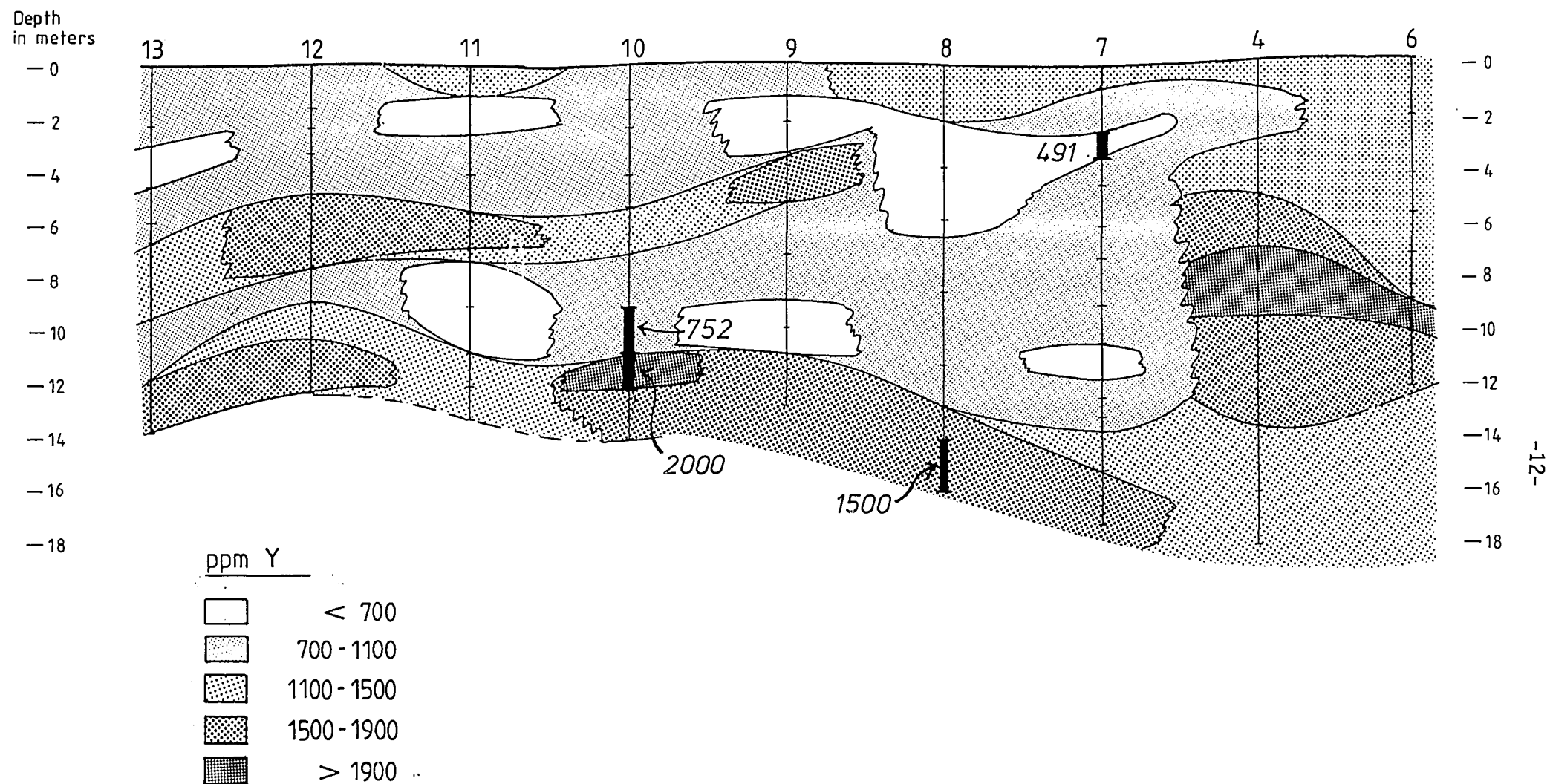
Fig. 3. Fordelingen av yttrium i Bordvedåga-forekomsten. De fire seksjonene hvor slip til mikrosondeundersøkelse er hentet fra er markert, og Y-innhold (i ppm) er påført.
