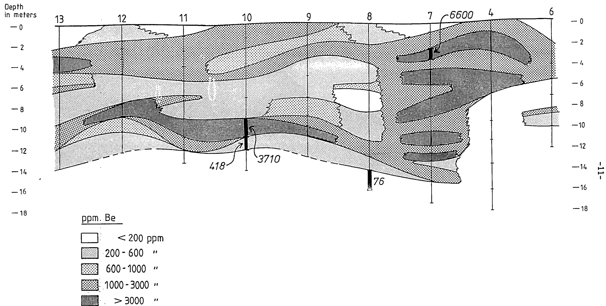
Fig. 2. Fordelingen av beryllium i Bordvedåga-forekomsten. De fire seksjonene hvor slip til mikrosondeundersøkelse er hentet fra er markert, og Be-innhold (i ppm) er påført.
