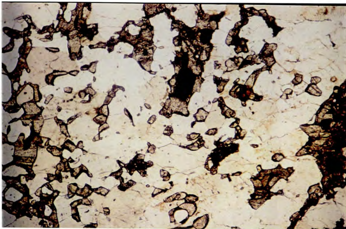
Fig. 43. Titanitt (lysebrun) i kvarts og feltspat. Biotitt er mørkebrun. Upolarisert lys. Skalastreken er 100 \mu m.
