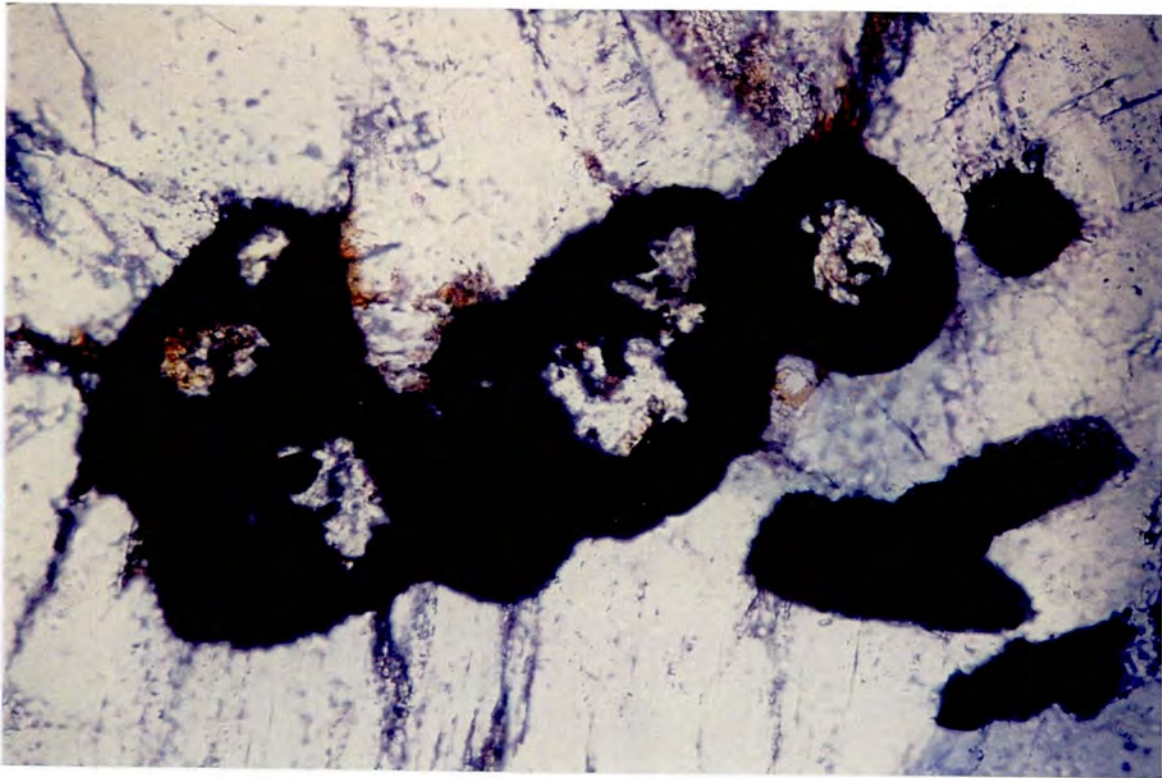
Fig. 66. Thoritt med magnetittrand. Upolarisert lys. Skalastreken er 100 \mu\text{m} .
