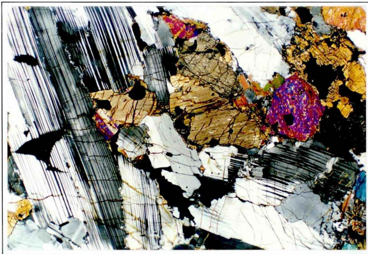
Figur 2. Tynnsnip av noritt fra prøvelokalitet 8 som viser fragmentering av plagioklasen og bøyde tvillinglameller.
