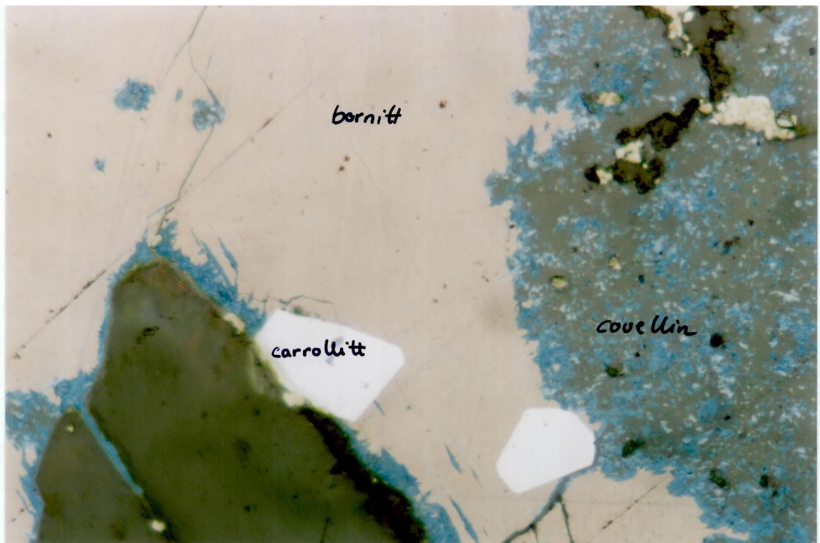
FIGUR 21: Euhedrale carrollitt-korn i bornitt som fortrenses av covellin og knapt synlige idattlameller i Skaudalen (slip 21995). Billedbredde 0.23 mm.
