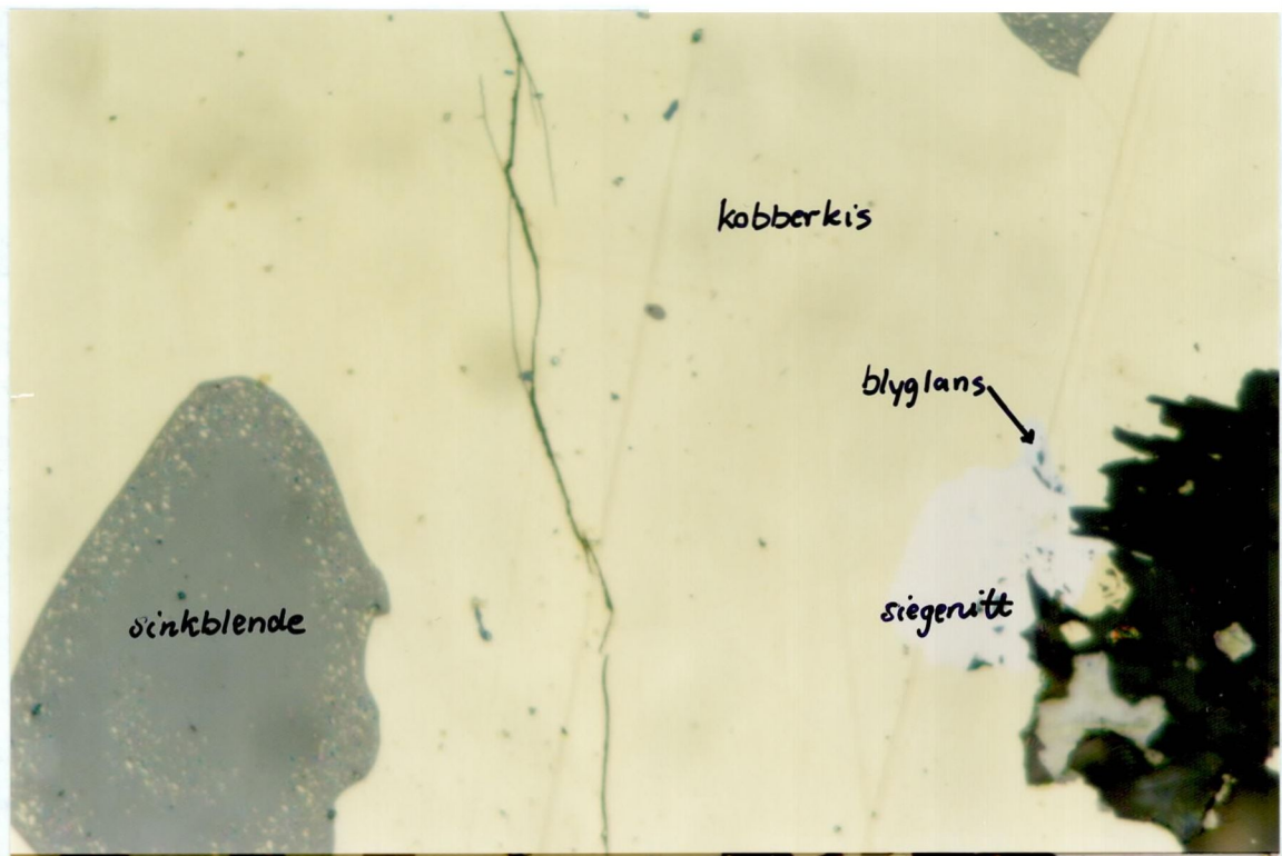
FIGUR 4: Euhedral siegenitt i kobberkis i Fines (slip 21988). Små inneslutninger av blyglans, og i tillegg sees skyer av ørsmå kobberkisinneslutninger i sinkblendens. Billedbredde 0.23 mm.
