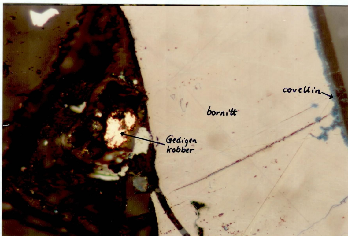
FIGUR 20: Uregelmessig korn av gedigen kobber nær bornitt i Skaudalen (slip 21995). Billedbredde 0.23 mm.
