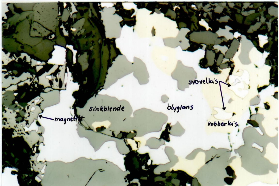
FIGUR 6: Bly- og sinkrik paragenese i Fines (slip 21985). Billedbredde 2.3 mm.
