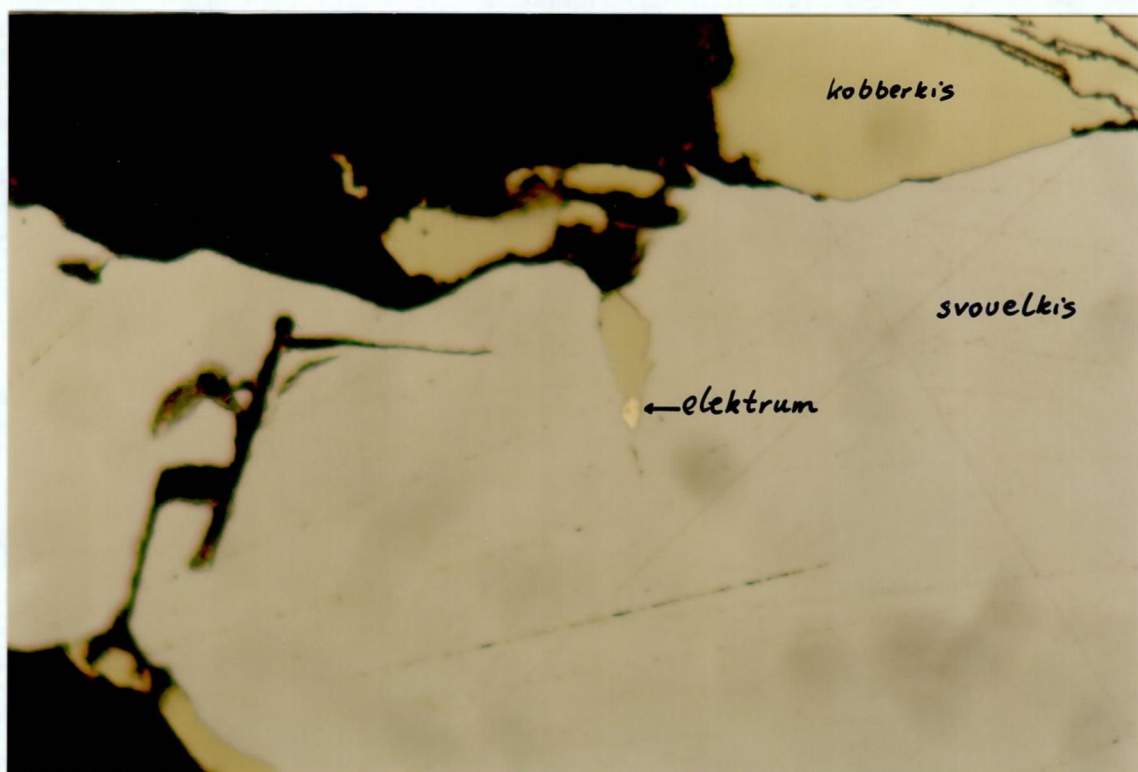
FIGUR 19: Elektrum-korn i kobberkis som trenger inn i svovelkis i Skaudalen (slip 9708). Billedbredde 0.23 mm.
