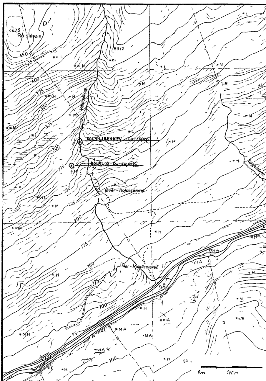
Figur 14: Rolslia og Rolslibekken skjerp.
