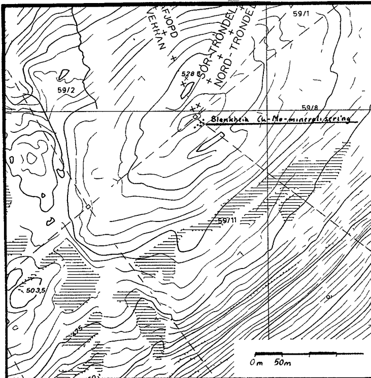
Figur 11: Blankheia mineralisering angitt ved prikker.
