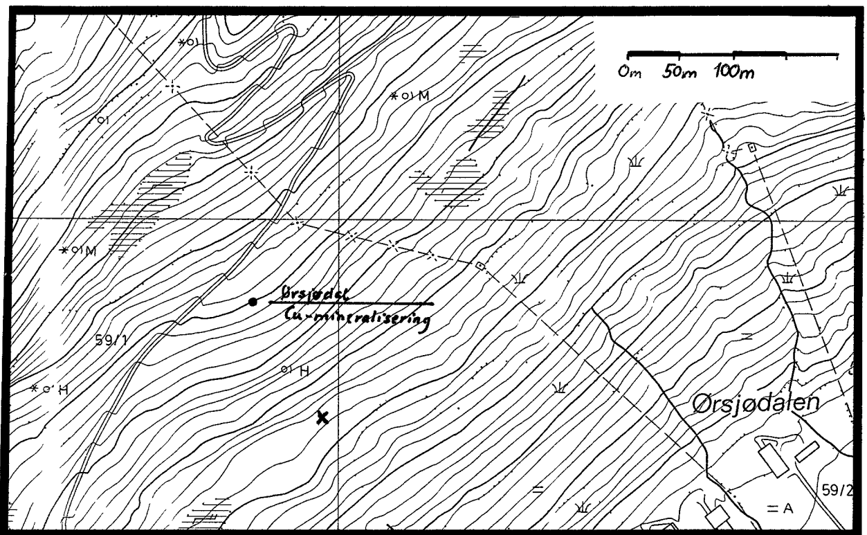
Figur 12: Kartet viser området rundt Ørsjødal "skjerp". Prikken angir prøvetakingssted, kryss angir en gråbergstipp.
