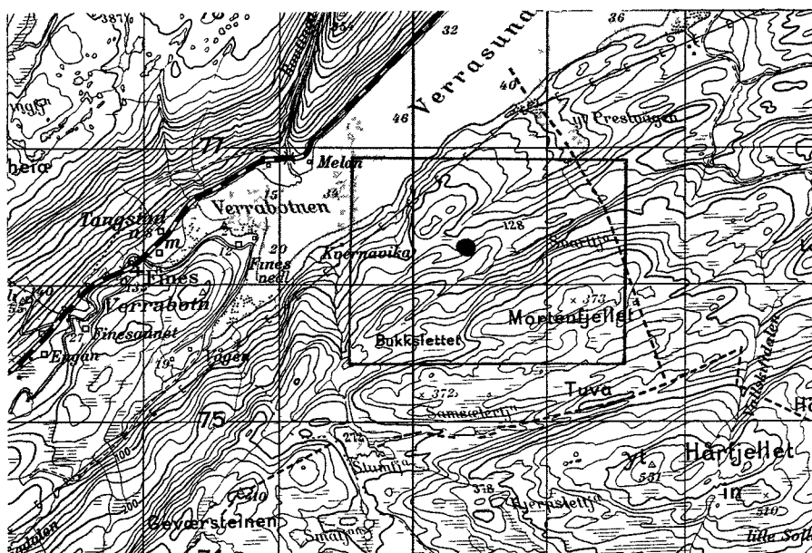
Figur 2: Lokalisering av Finesgruva (prikk) (M 1:50000).
