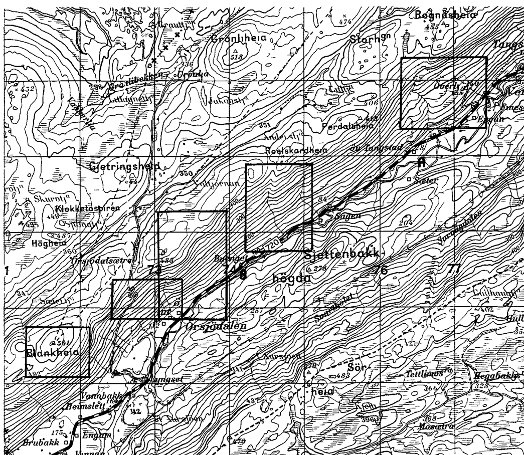
FIGUR 10: Lokalisering av malmforekomstene i Ørsjødalen. Rektangel nr. 1 (til venstre) omfatter Blankheia, nr. 2 viser Ørsjødal, nr. 3 Kamberga og Buengheia, nr. 4 Rolslia og Rolslibekken og nr 5 Svartbekken. Rektanglene representerer kartene i figur 11-15. "A" og "B" viser plassering av påståtte mineraliseringer (kommenteres i tekst). (M 1:50000)
