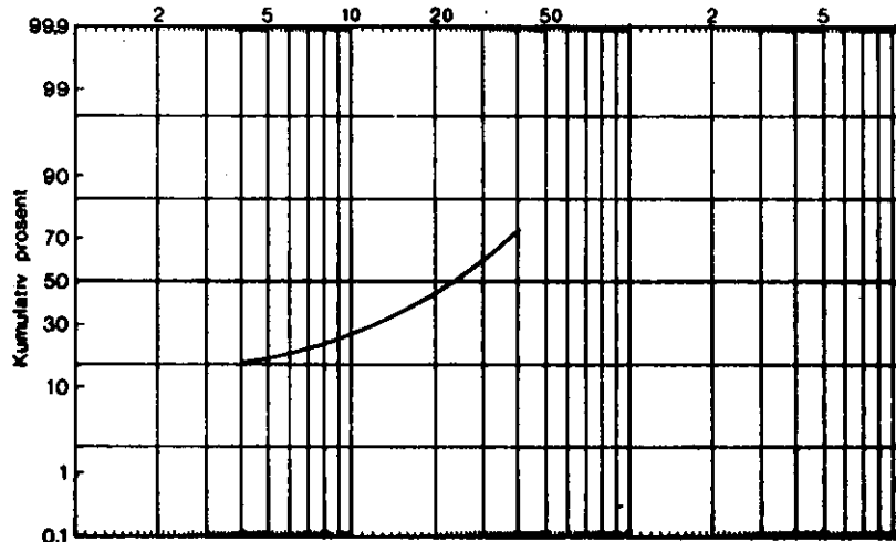
FREKVENSFORDELINGSDIAGRAM PÅ FORHOLDET MELLOM MgO/SiO 2 . BASERT PÅ 50 PRØVER
