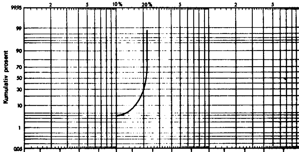
FREKVENSFORDELINGSDIAGRAM PÅ MgO. BASERT PÅ 46 PRØVER
