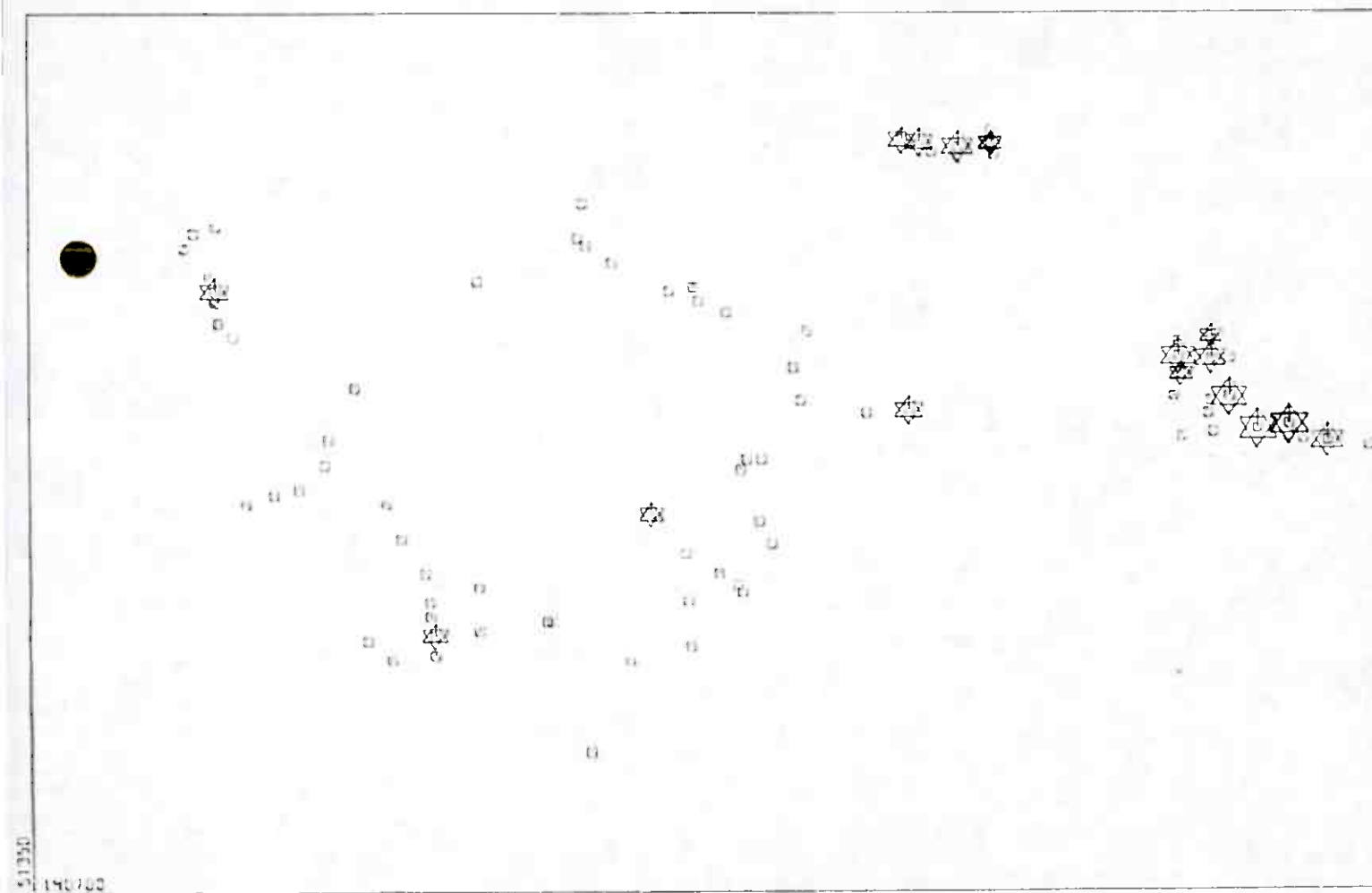
Fig. 10 VIPETO-RULLENOLL AREA • THORIUM • STAR IF Z > 0.05 MAP
