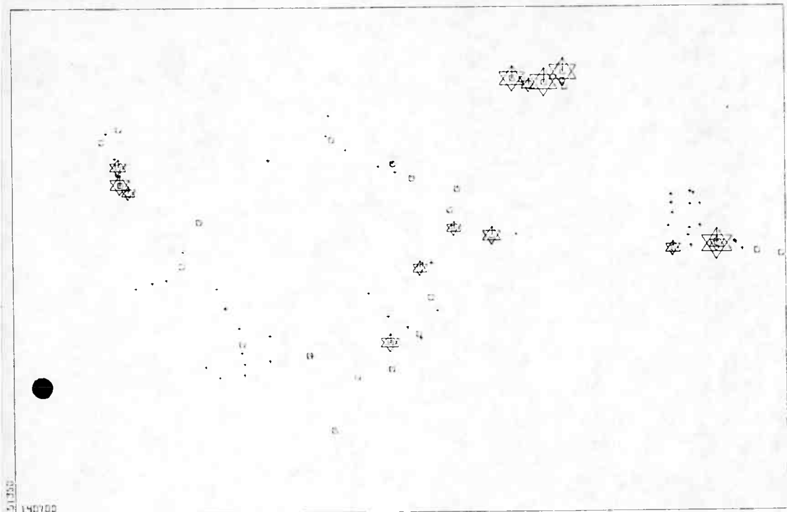
Fig. 9 VIPETO-RULLENOLL AREA • BARIUM • STAR IF Z > 0.5 MAP
