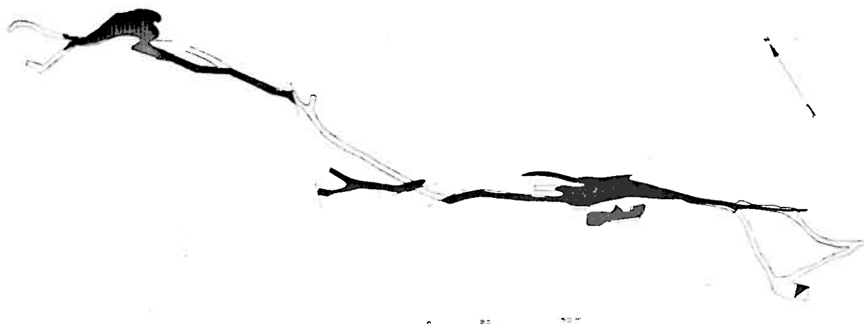
Fig. 4. Horizontalschnitt der 160 m-Sohle in der Alten Vigsnes-Grube. Nach einem alten Grubenriss. Die Erzkörper zeigen die für viele Kieslagerstätten typische gestaffelte Anordnung.
