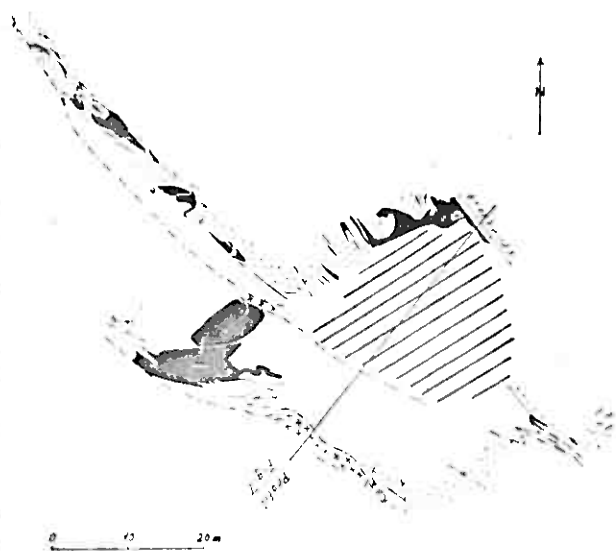
Fig. 6. Rökklev-Grube. Horizontalschnitt der 280 m-Sohle im Ostkies. Schraffiert: abgebaute vererzte Partien, Zeichenerklärung s. Fig. 7. Situation 1958.
