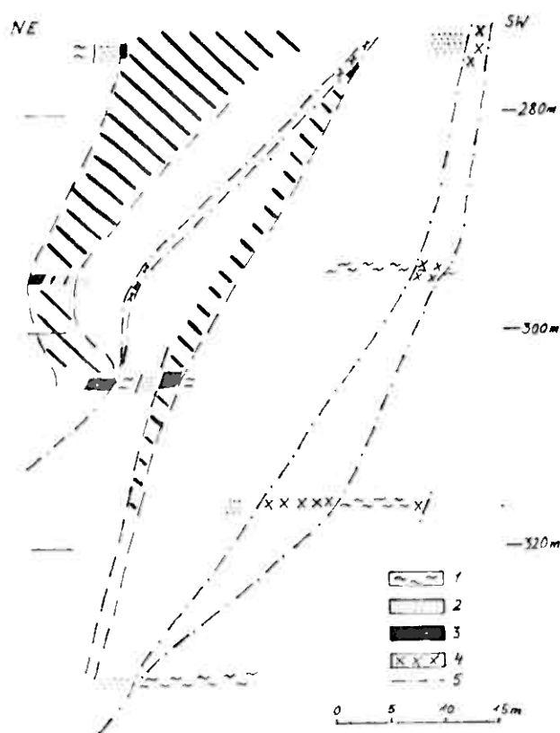
Fig. 7. Rødklev-Grube. Profil durch den unteren Teil des Ostkieses. Schuftiert, abgebaute verzte Partien. Situation 1958.
