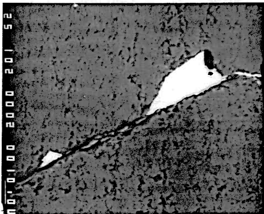
Fig. 2: Backscatter bilde med ged. vismut (hvit) i en sprekk i pyritt (grå). Bildet er en utsnittsforstørrelse av Fig. 1. 1000 x forst.
