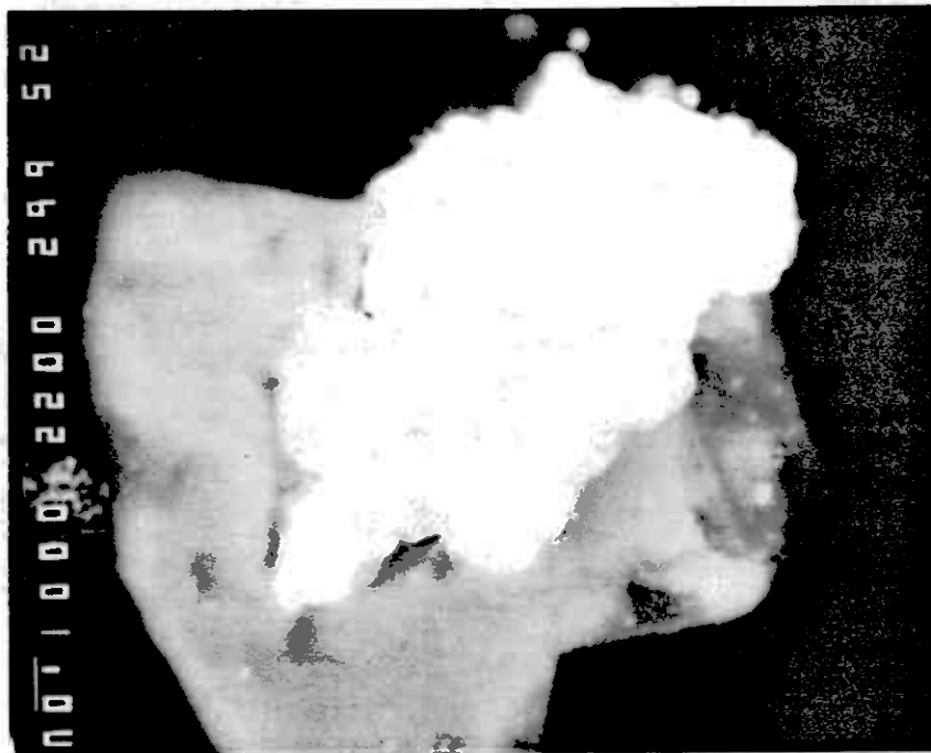
Fig. 15: Backscatter bilde av Th-holdig uraninit (hvit) i pyritt (grå). Mellom uraninit og pyritt er en tredje fase. Amfibol er mørkt. 6600 x forstørrelse.
