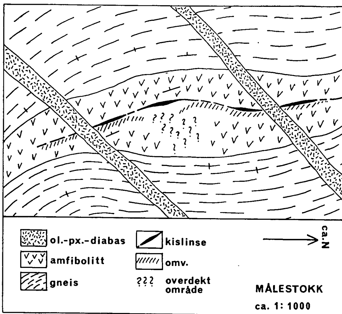
Fig. 3.1 Skisse over gruveområdet ved Haugset gruve.
