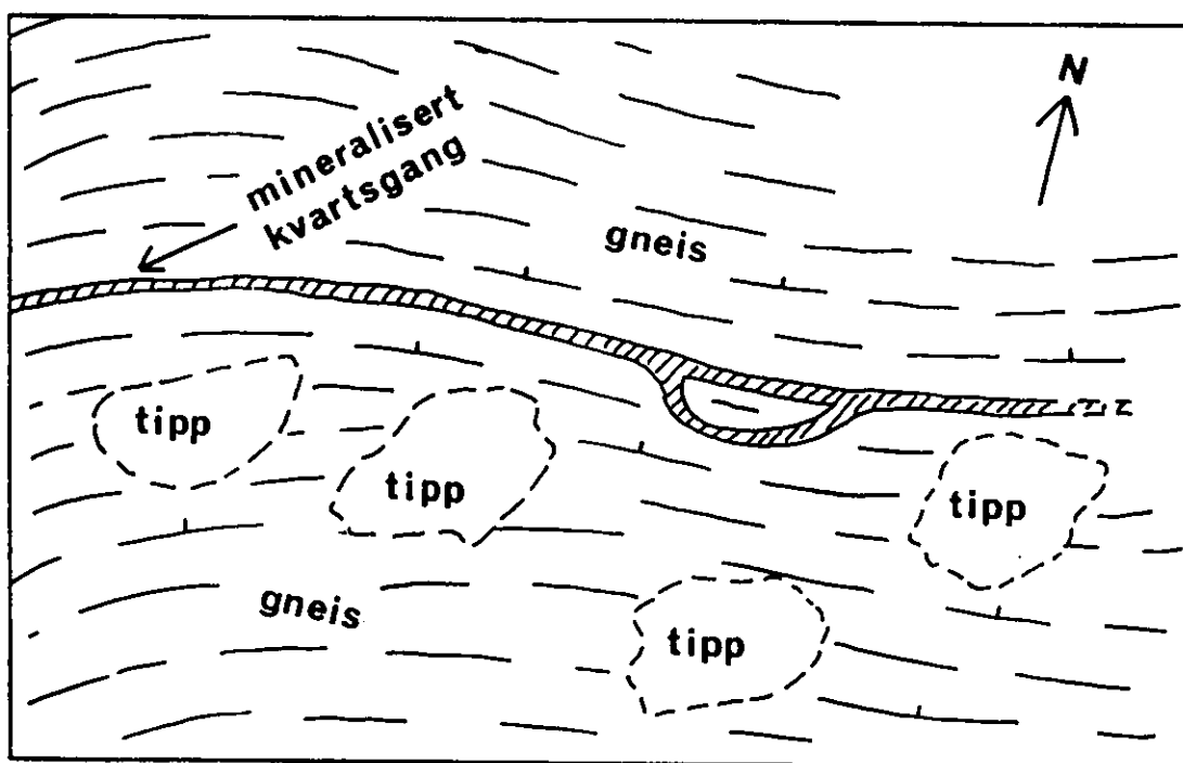
Fig. 3.2. viser en skisse over Åsgruva. (Målestokk ca. 1:1000)
