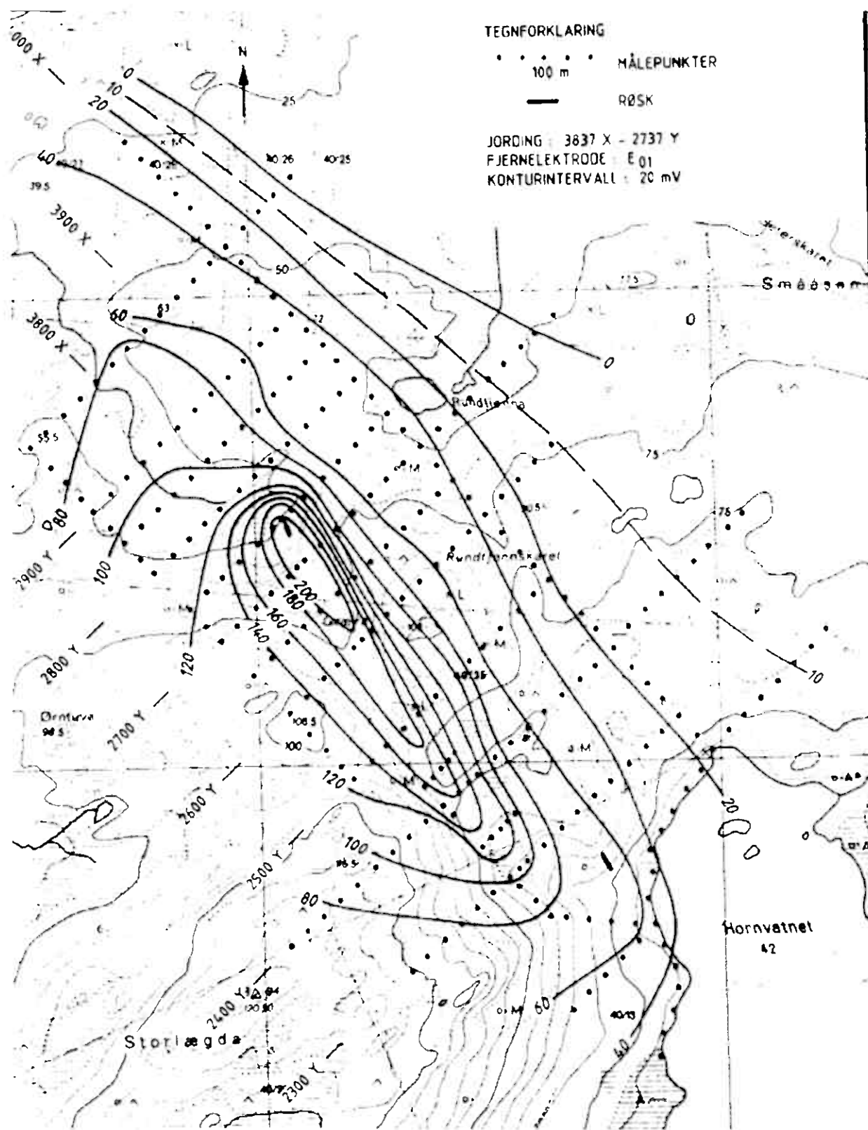
Figur 3CP anomalikart over Græva malmkropp
