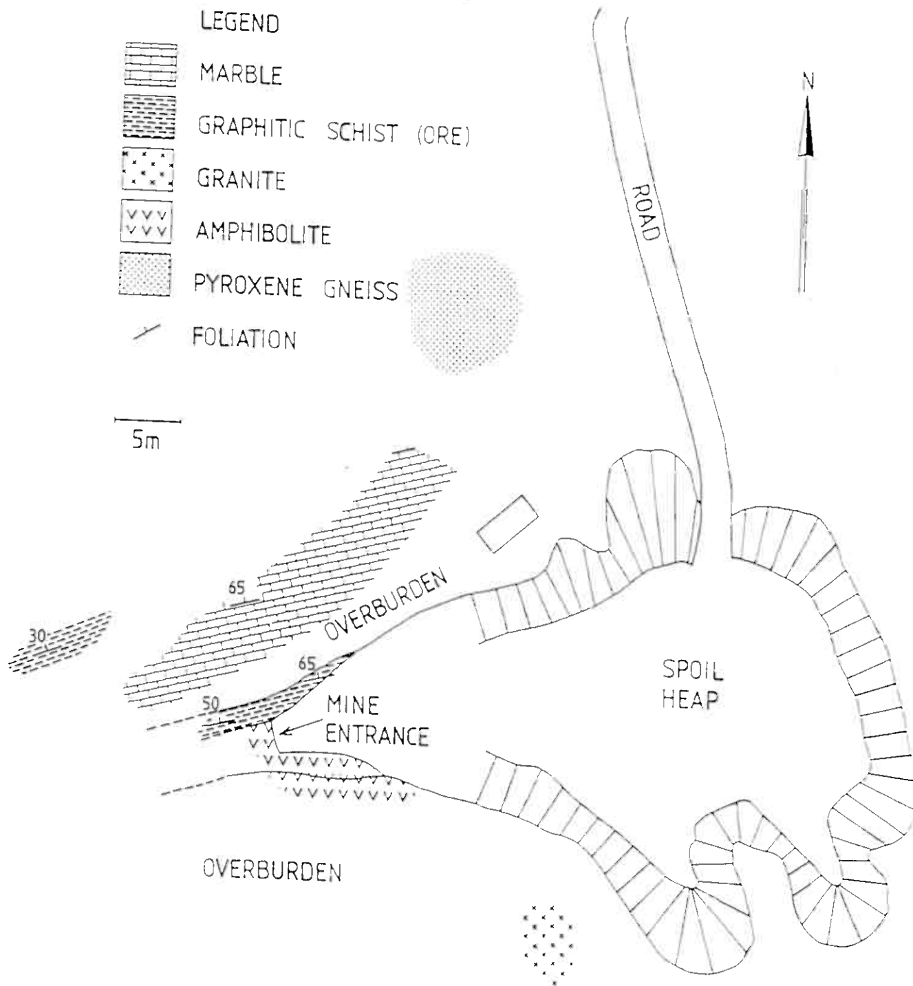
Figur 2 Detaljkart over Golia
