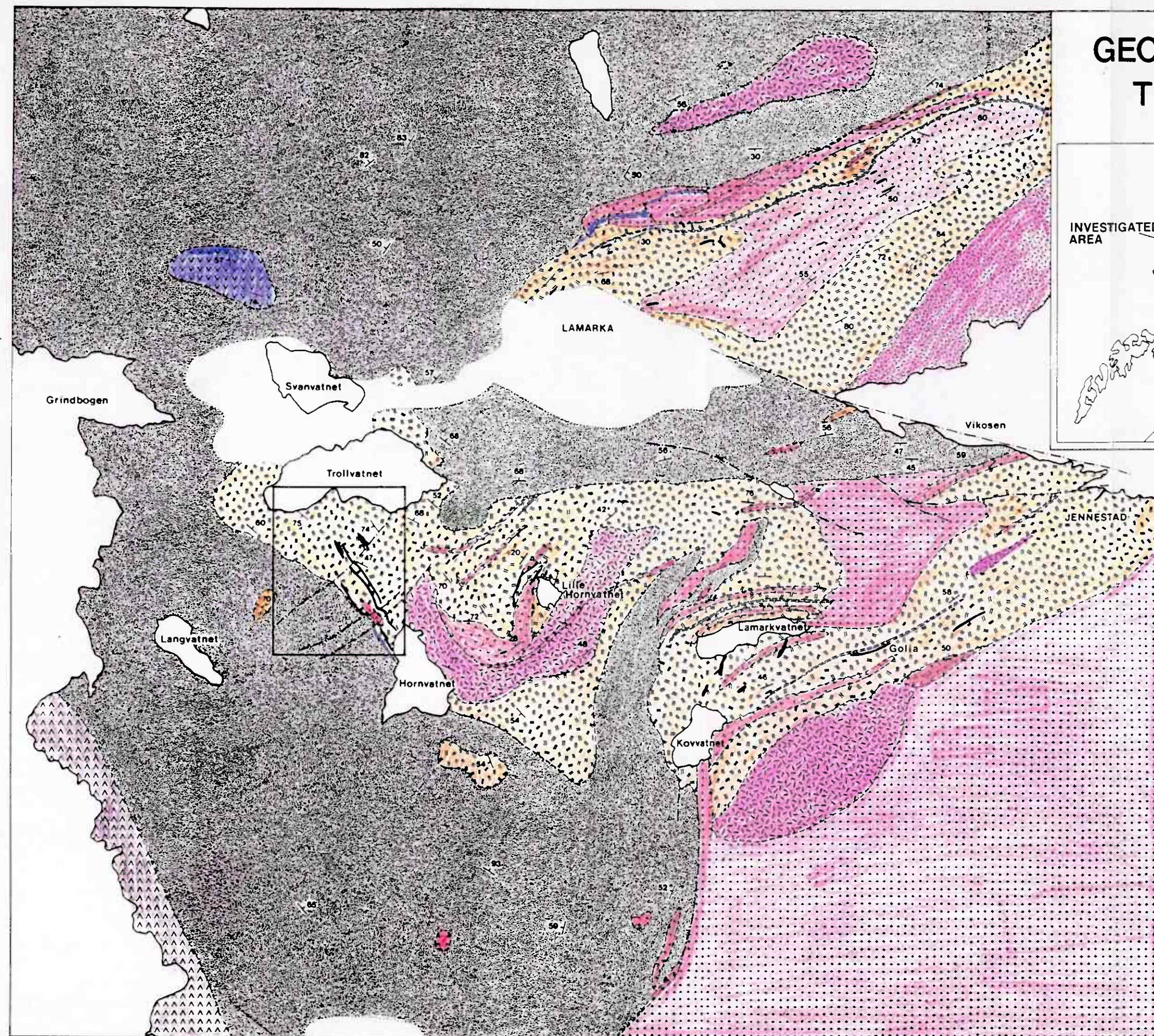
Figur 1 Geologisk kart over Vikeidområdet
