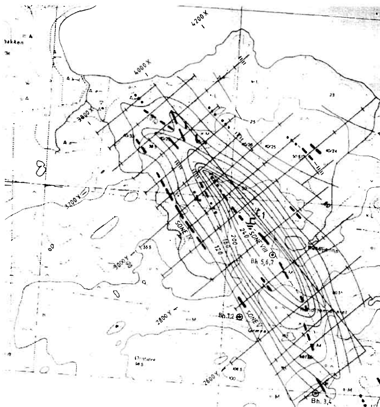
Figur 5 CP anomalikart over Rundtjernmalmkropp
