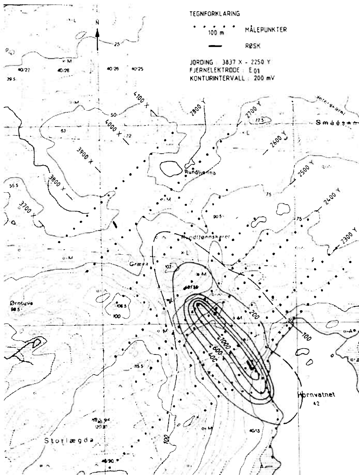
Figur 4 CP anomalier over Hornvannet malmkropp (Rønning 1991)
