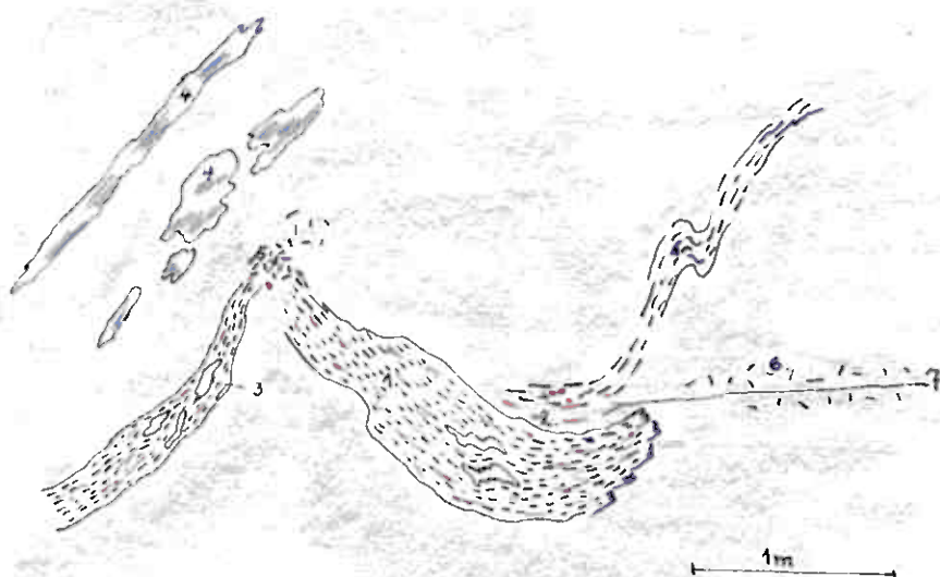
Fig. 6. Detalj som viser både grønnsten og malin involvert i folding. Skisse 31
