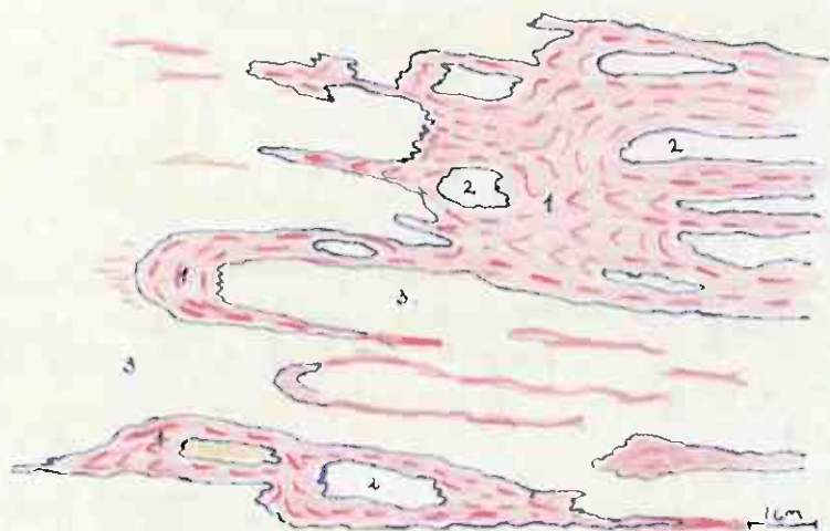
Fig. 2. Isoklinalt foldet malm streiper ved enden av '2:7-malmen' (pr. 63)
