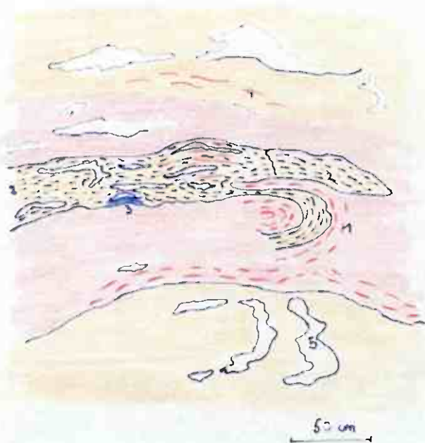
Fig 4 Foldet malm og grønnsten, angitt på 10,0 - 11,5 m over lotte
