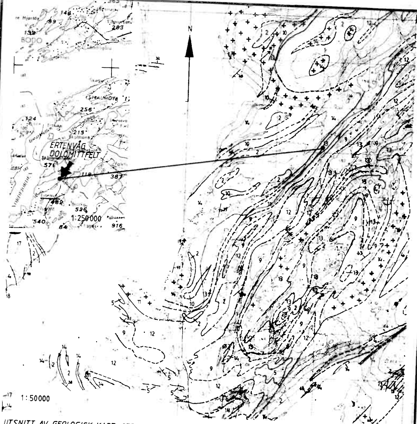
UTSNITT AV GEOLOGISK KART: STRØMØEN 1:50000 AV A.SOLLI
