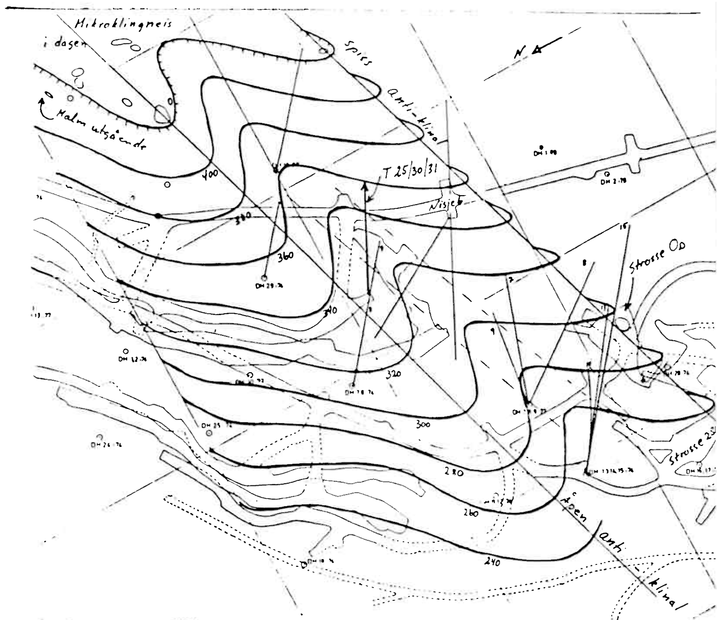
Fig. 5. Intenst foldet parti mellom Nordmalmen (venstre) og Hovedmalmen anskueliggjort med koter i heng av mikroklingneis som ligger like under malmensonen. Strukturen innledes med en åpen antyklinal, fulgt av en kompleks synklinal (forenklet) og en spiss, høy antyklinal. Rik malm er drevet ut i deler av synklinal ved 320 og i strosse 250, samt påtruffet i det mellomliggende parti i DH 7/77.
