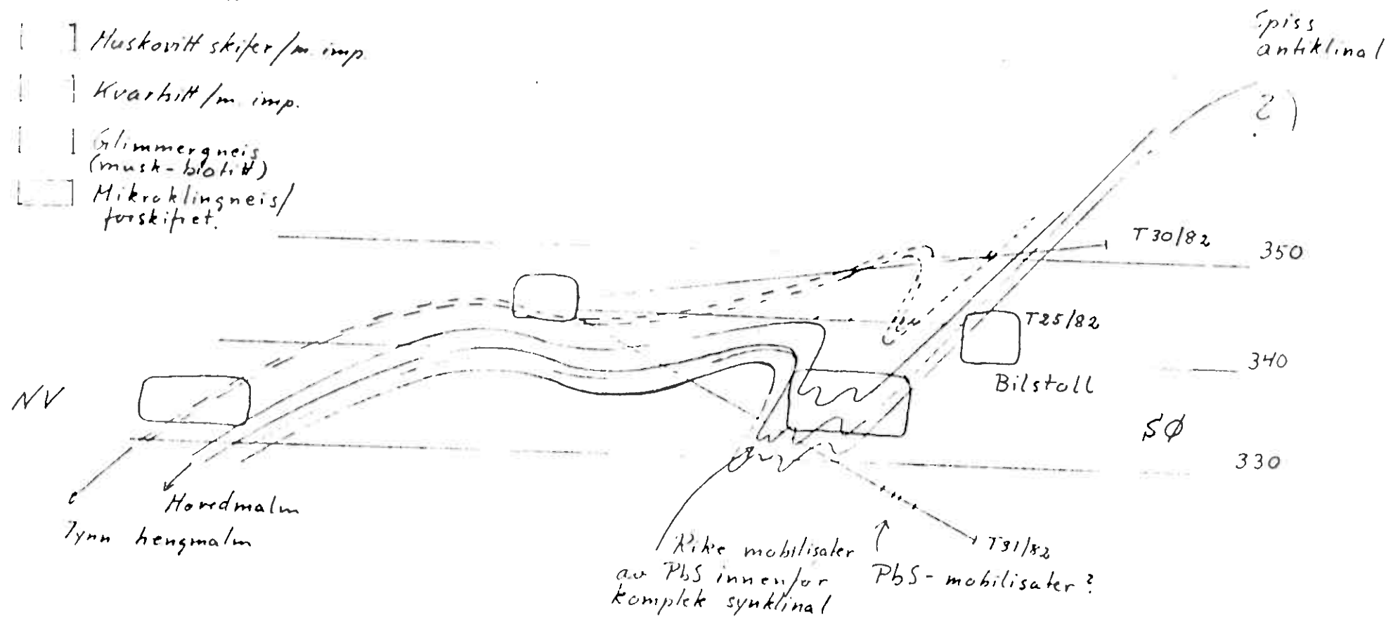
Fig. 6: Foldefortykkelser og mobilisater av malm i kompleks synklinal. Boreprofil nivå 340 S, profilretning N 120° Ø, målestokk 1: 500. Malm oppover i vestflanken av "spiss antyklinal" synes gradvis å bli svakere. Malm er også påvist rett under nisje 6 (litt syd for profilet) som antas å ligge i en posisjon som tilsvarer østflanken av samme spisse antyklinal.
