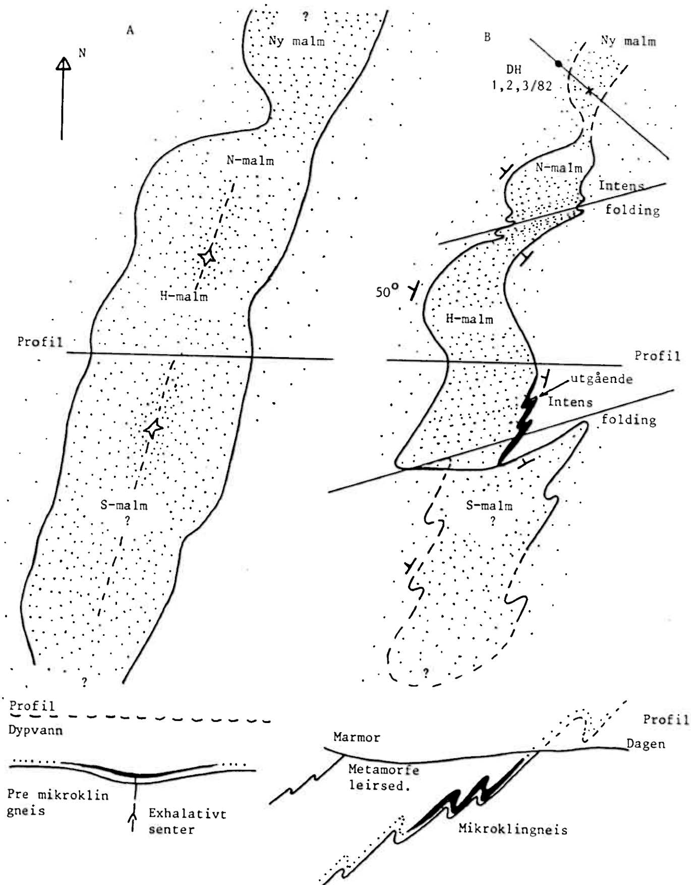
Fig. 2 : Modell for Bleikvasslimalmen : A) Primært langstrakt avsetningsbasseng med tenkte exhalative sentra (stjerne).
