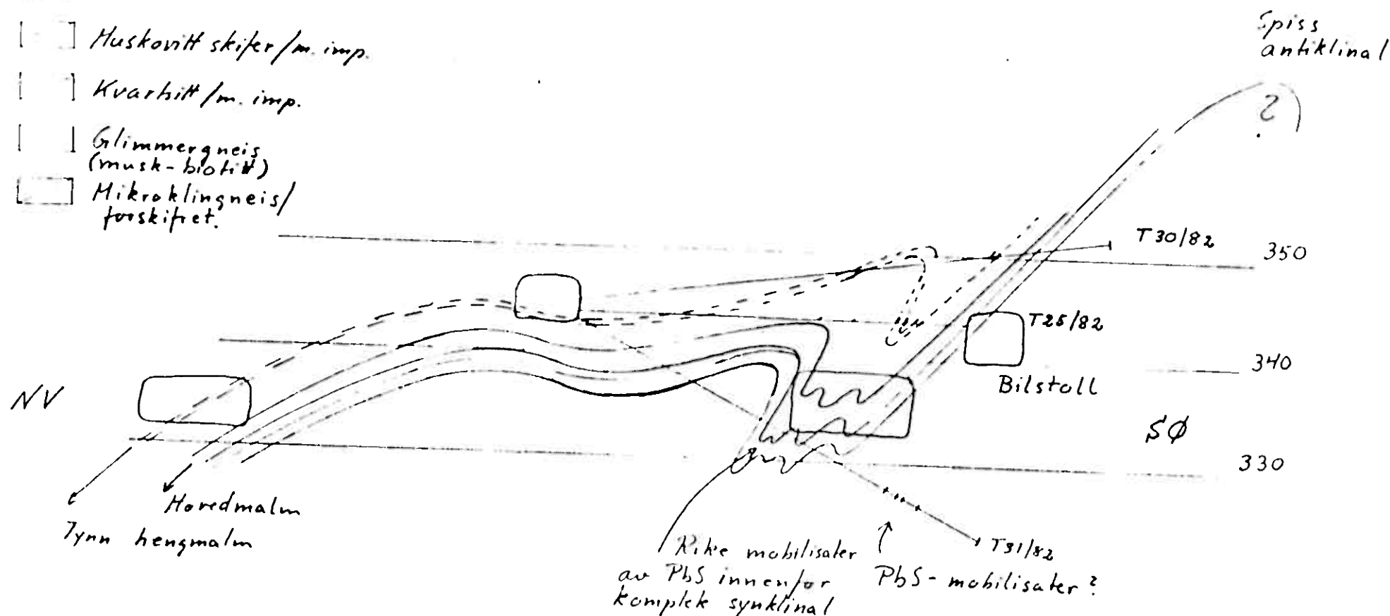
Fig. 6: Foldefortykkelser og mobilisater av malm i kompleks synklinal. Boreprofil nivå 340 S, profilretning N 120° Ø, målestokk 1: 500. Malm oppover i vestflanken av "spiss antiklinal" synes gradvis å bli svakere. Malm er også påvist rett under nisje 6 (litt syd for profilet) som antas å ligge i en posisjon som tilsvarer østflanken av samme spisse antiklinal.
