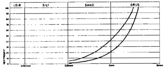
Dekker av olje og asfaltløsningsgrus
