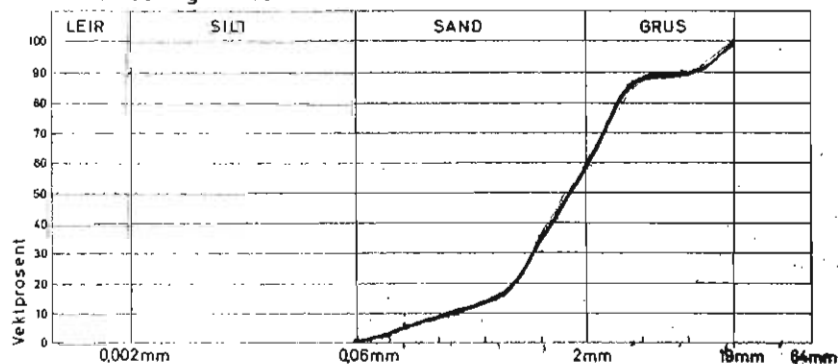
Kornfordelingskurve
