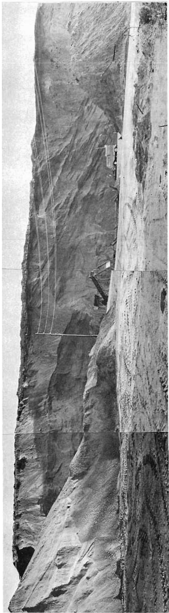
Fig. 1: Ålmo massetak. Borhull 1 ligger bak bilen.
