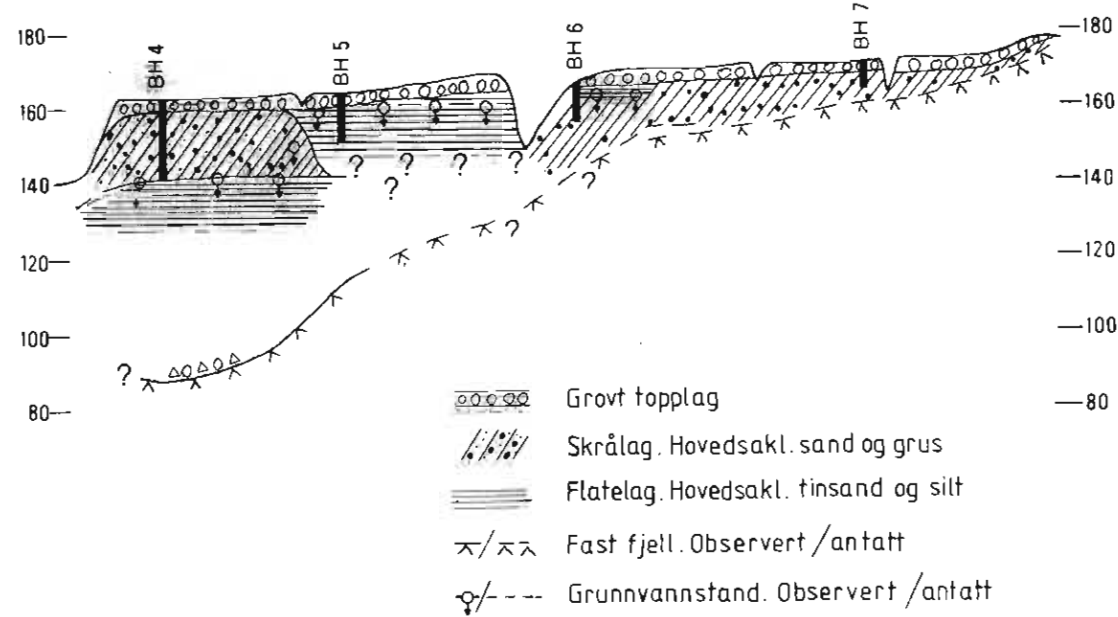
SKROMOTERASSEN, Skjematisk løsmasseprofil Forventet fordeling og oppbygging av løsmassene
