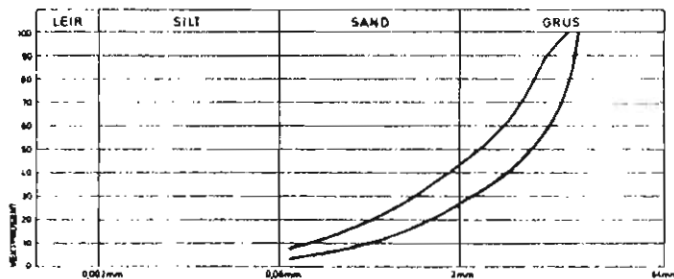
Asfaltgrusbetongdekker (Agb 16)
