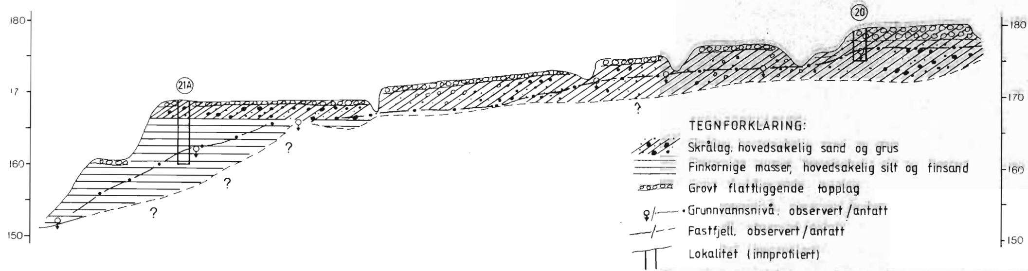
SNÅSAHEIA. Skjematisk løsmasseprofil. Forventet fordeling og oppbygning av løsmassene.
