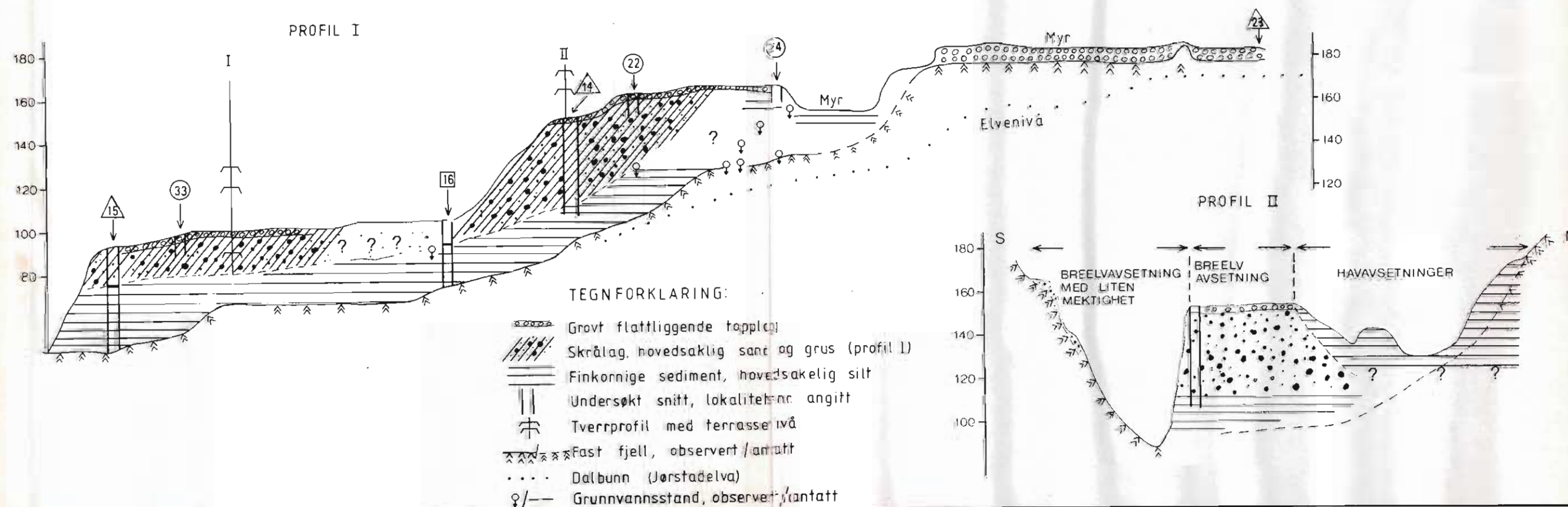
KJENDSTADAVSETNINGEN. Skjematisk løsmasseprofil. Forventet fordeling og oppbygning av løsmassene.
