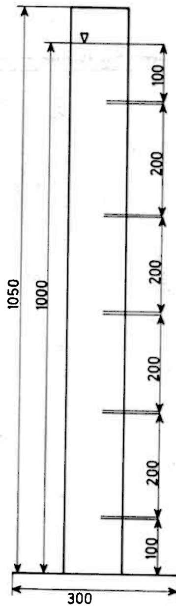
Fig. 5 Longtube for måling av sedimentasjonshastighet Mål i mm
