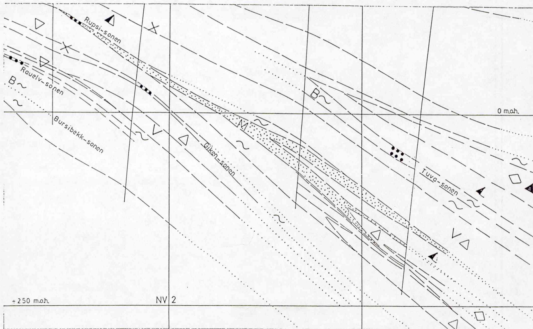
Fig. 7.11. Rupsifeltets kisser, bl.a. med Rupsi-forekomsten. Utsnitt fra profil NØ-6 i målestokk 1:2.500
