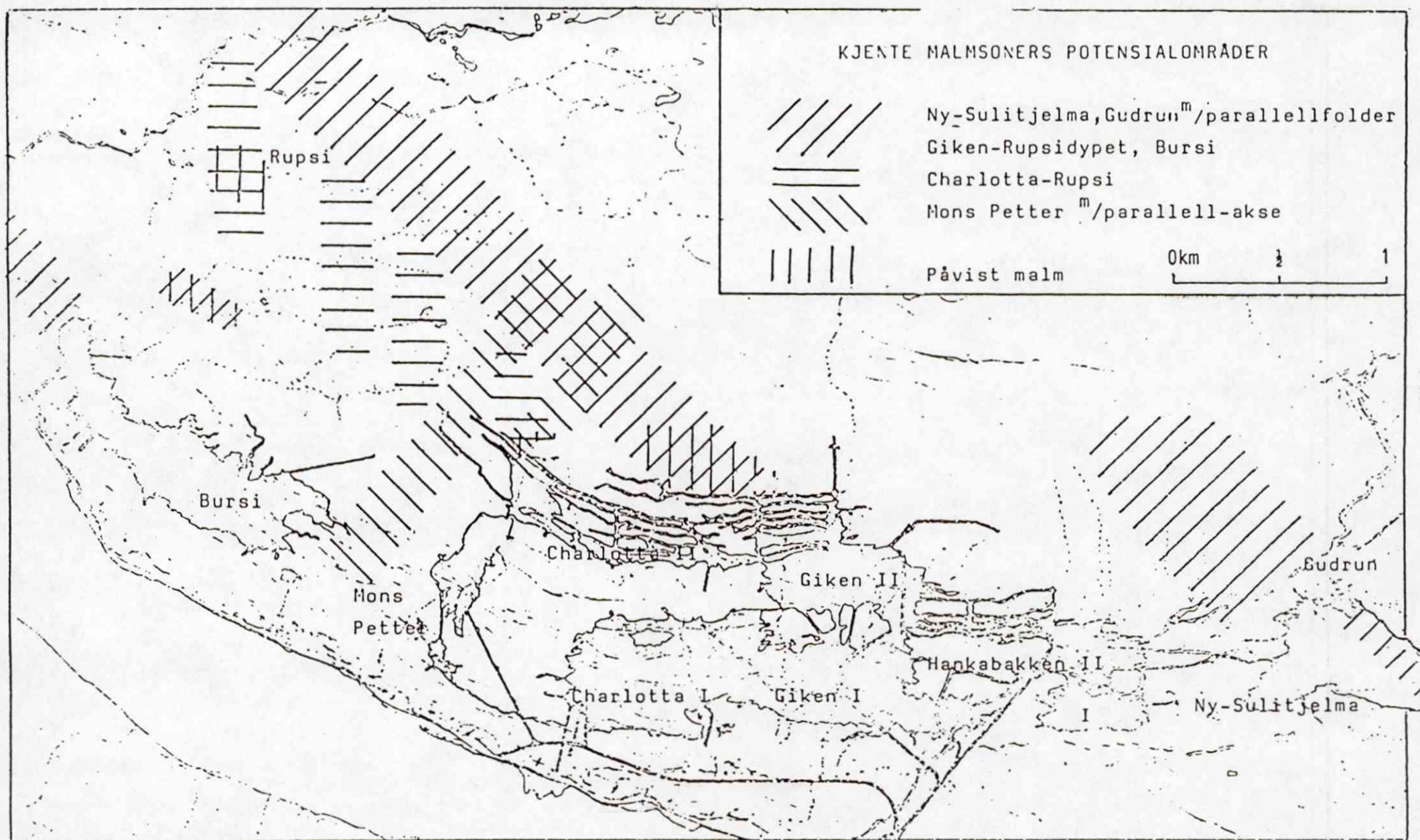
Fig. 8.13. Antydnet område for potensielle malmer tilknyttet kjente malmsoner i Nordgruvefeltet.
