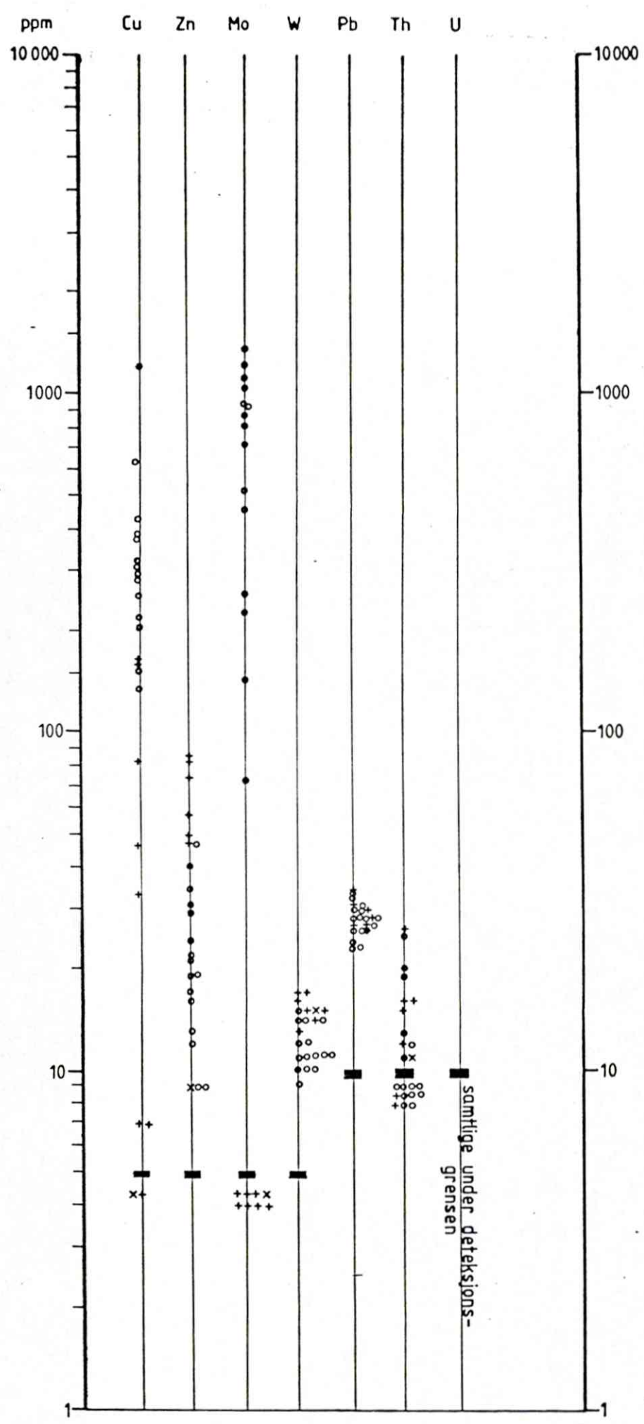
Fig. 10: Spor-elementer i bergartsprøver fra Amlandsheia.
