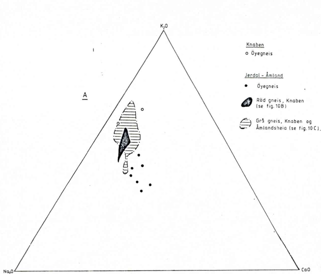
Fig.9: Trekantsdiagrammer for forholdene mellom \text{Na}_2\text{O} - \text{K}_2\text{O} - \text{CaO} i de forskjellige bergartstypene på Åmlandsheia og fra Knaben.
