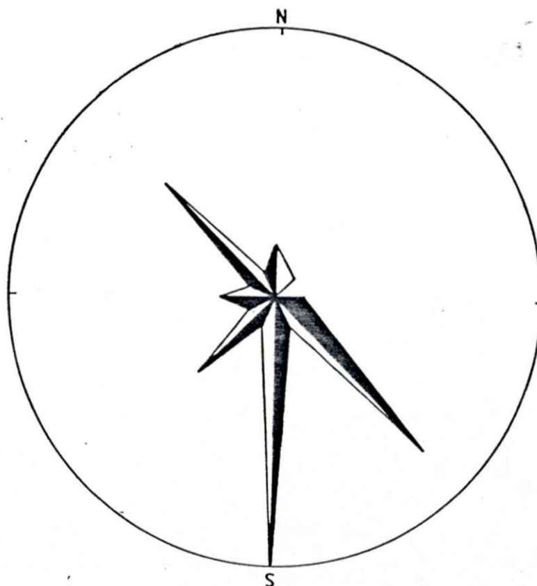
Fig. 4: Rosediagram av observerte sprekkeretninger i felt. Frekvensen innenfor 50 g intervaller, ialt 16 målinger.
