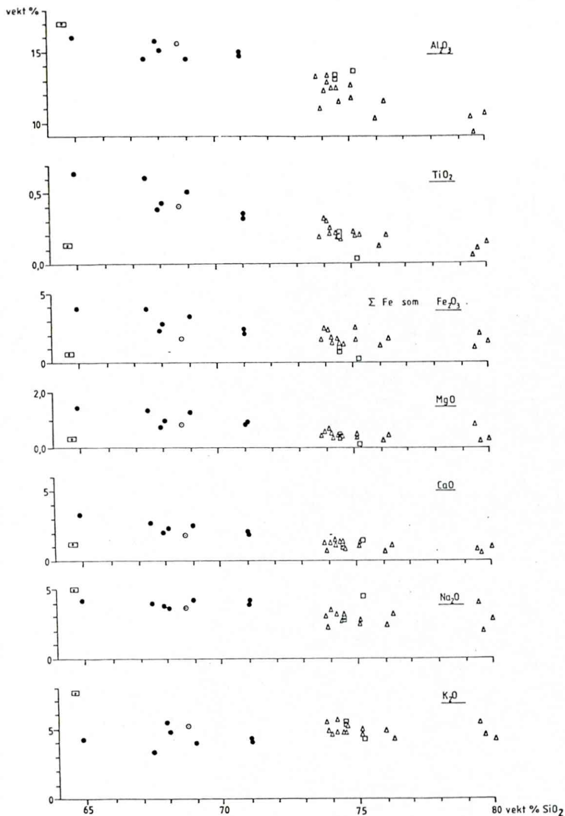
Fig. 7: Kjemiske analyser av hovedelementene fra 24 bergartsprøver gjengitt i et Harkers-variasjonsdiagram. Lukkede sirkler : øyegneis, trekanter : granittisk gneis, firkant : pegmatitt. Tre analyser fra Knaben II, vertikal rektangel : aplitt gang, horisontal rektangel : gangfjell.
