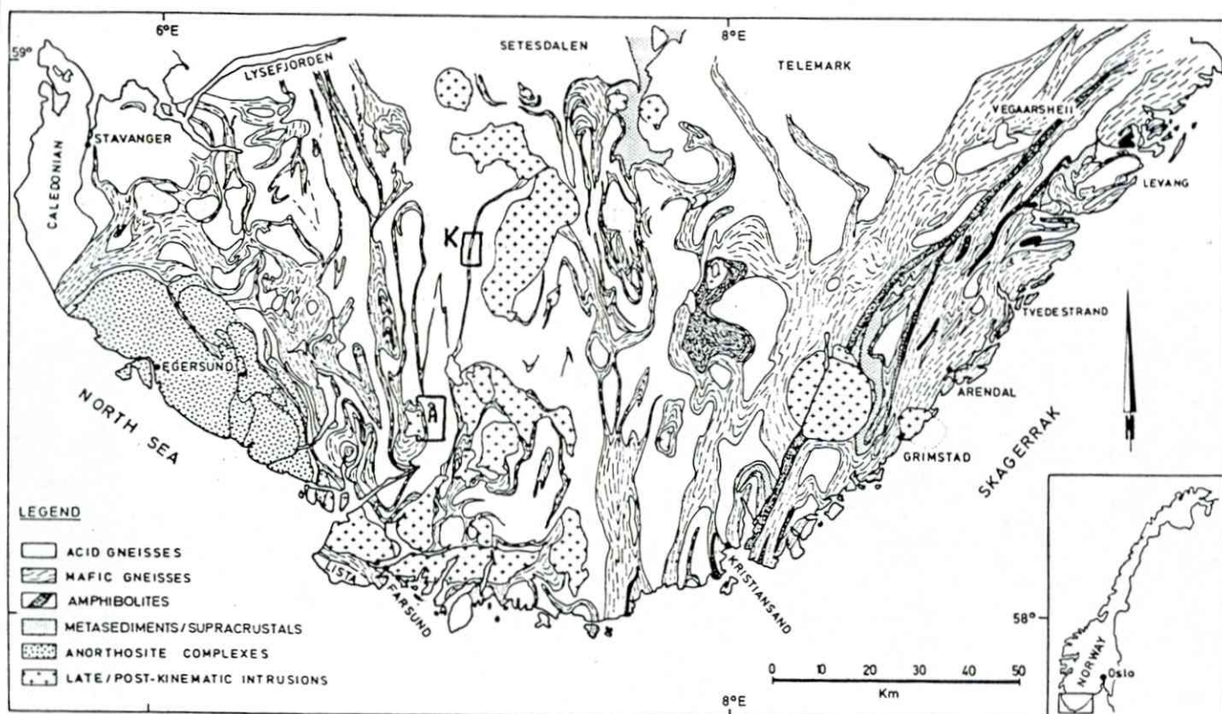
Fig. 1 Geologisk kartskisse over Sør-Norge med de viktigste lithologiske enhetene (kopi fra Falkum & Petersen 1980, fig. 1).
