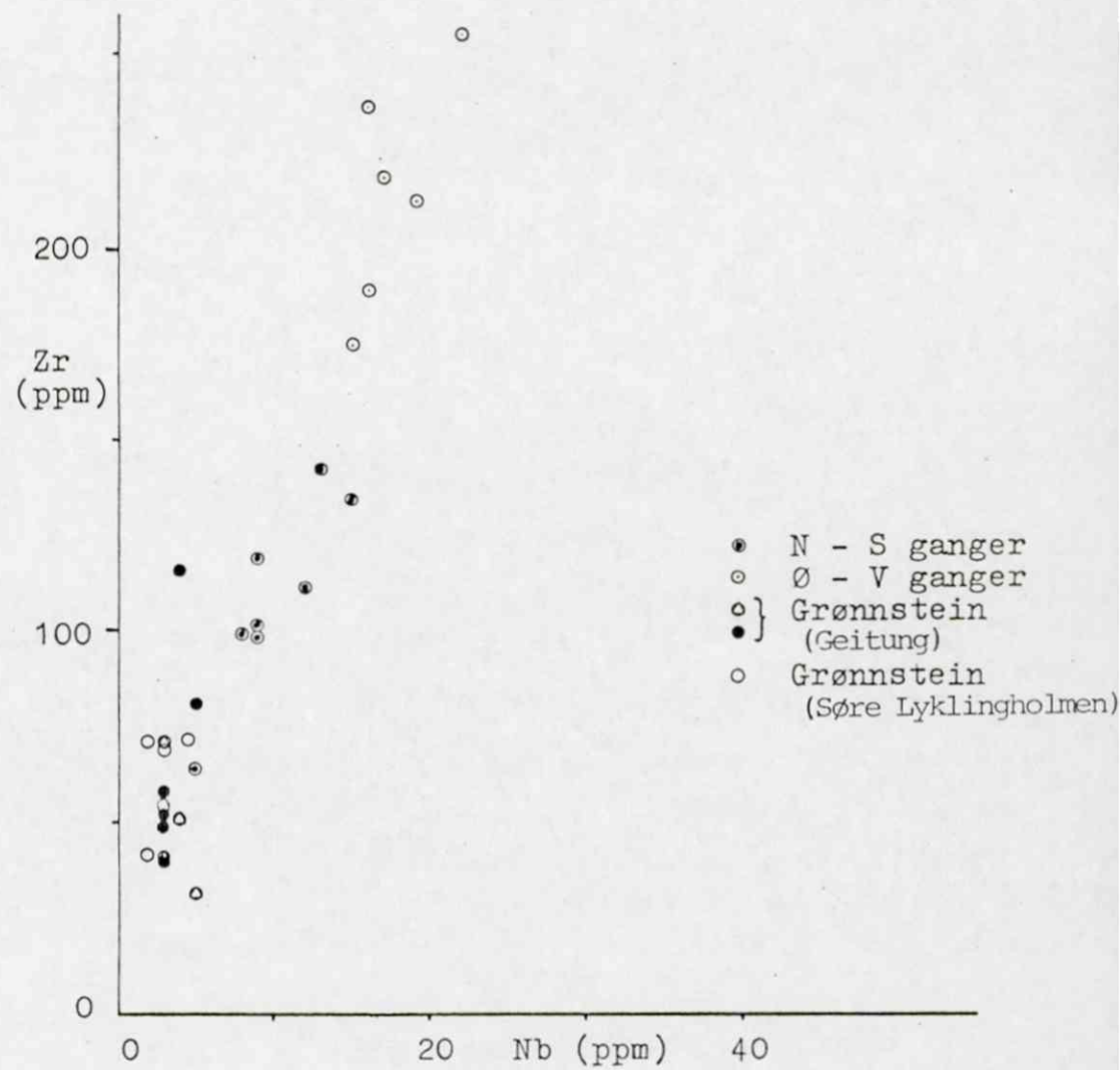
Fig. 7. Zr/Y og Zr/Nb plot fra dolerittiske ganger og fra ophiolitt grønnstein.
