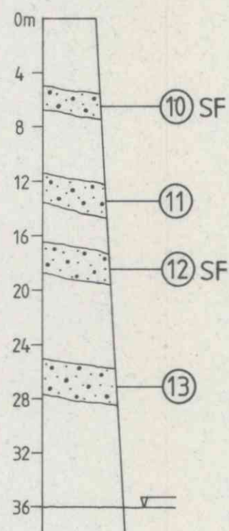
Snitt C
