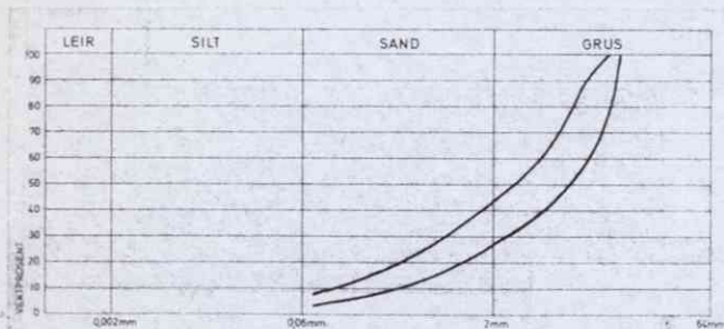
Asfaltgrusbetongdekker (Agb 16)
