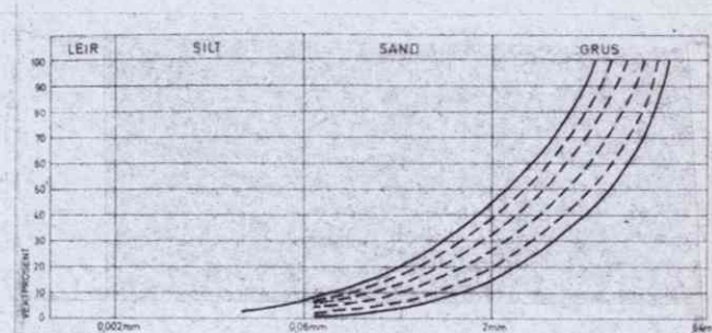
Bærelag
