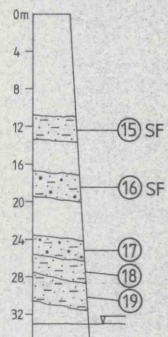
Snitt E
