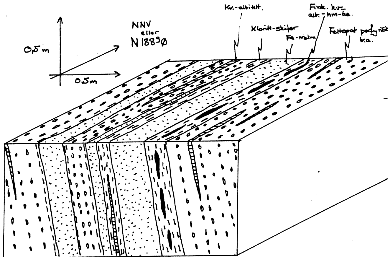
Fig. 5. Skjematisk profil av malmsonen i nordre del av Føskerseter gruve.
